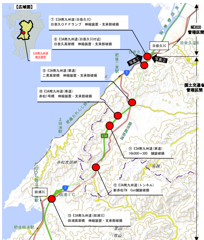
①被災状況（伸縮装置破損）
