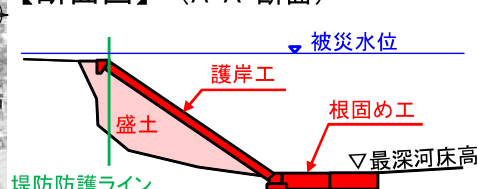
【断面図】 (A-A'断面)
