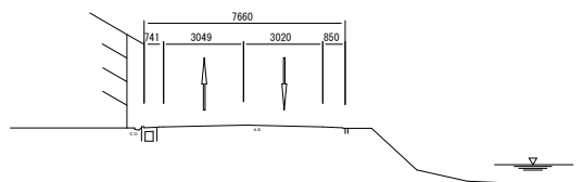
【横断図】
