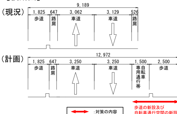
【横断図】
