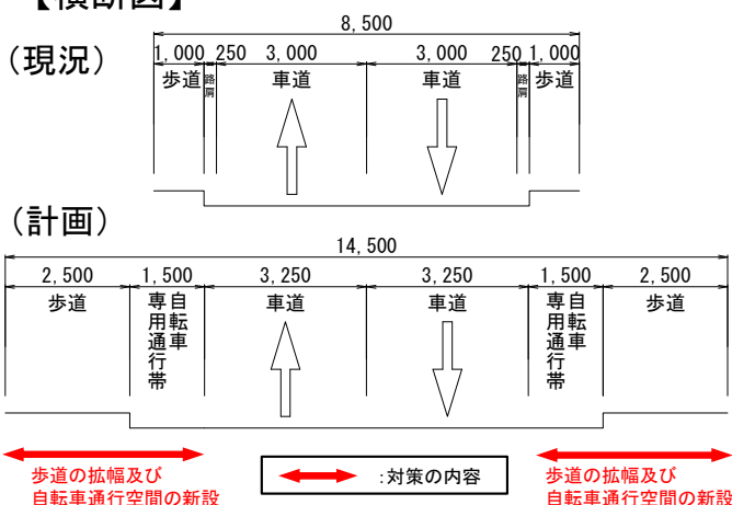
【横断図】
