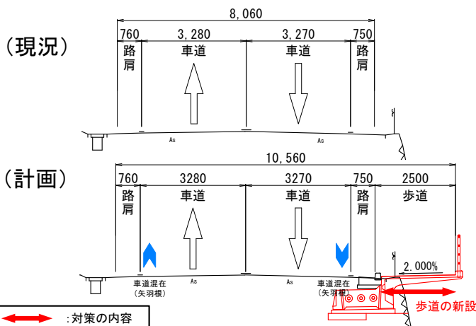
【横断図】(黒岩地区)
