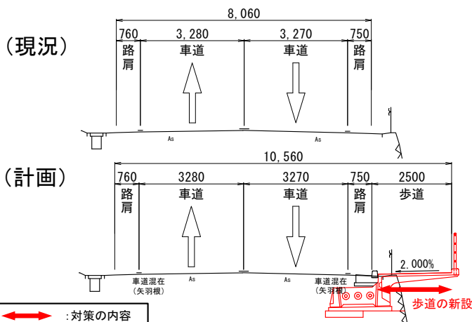
【横断図】（黒岩地区）
