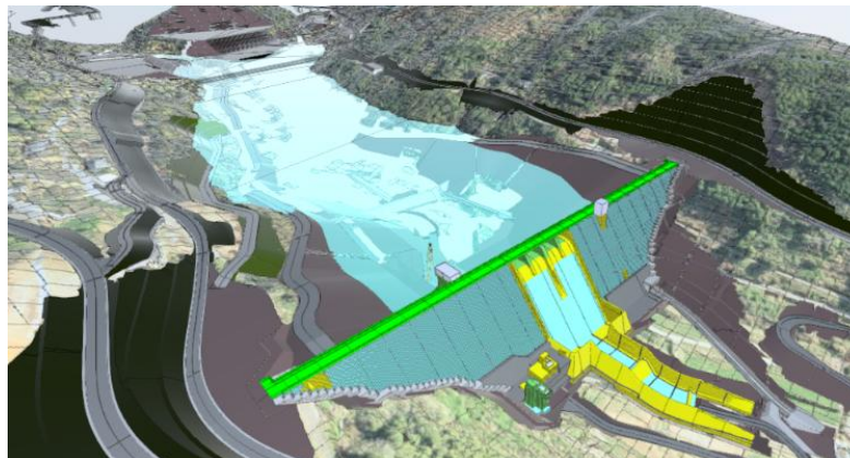
⑥完成【常時満水位】(R14)
