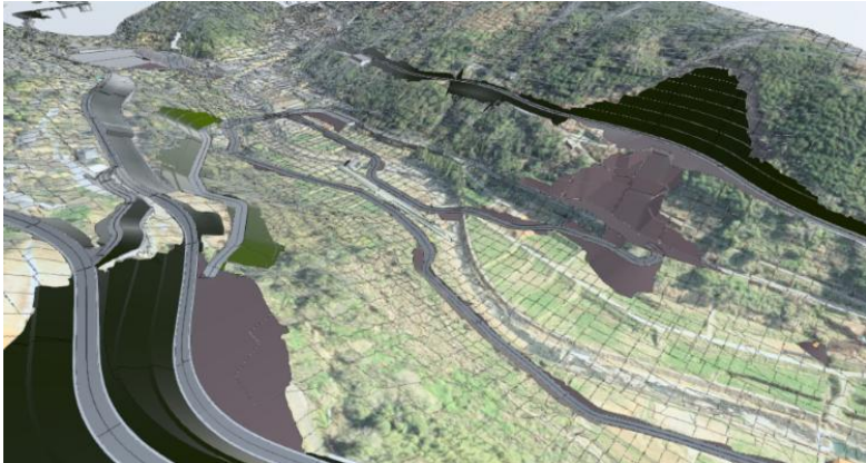
③CSG打設 (R10～)
