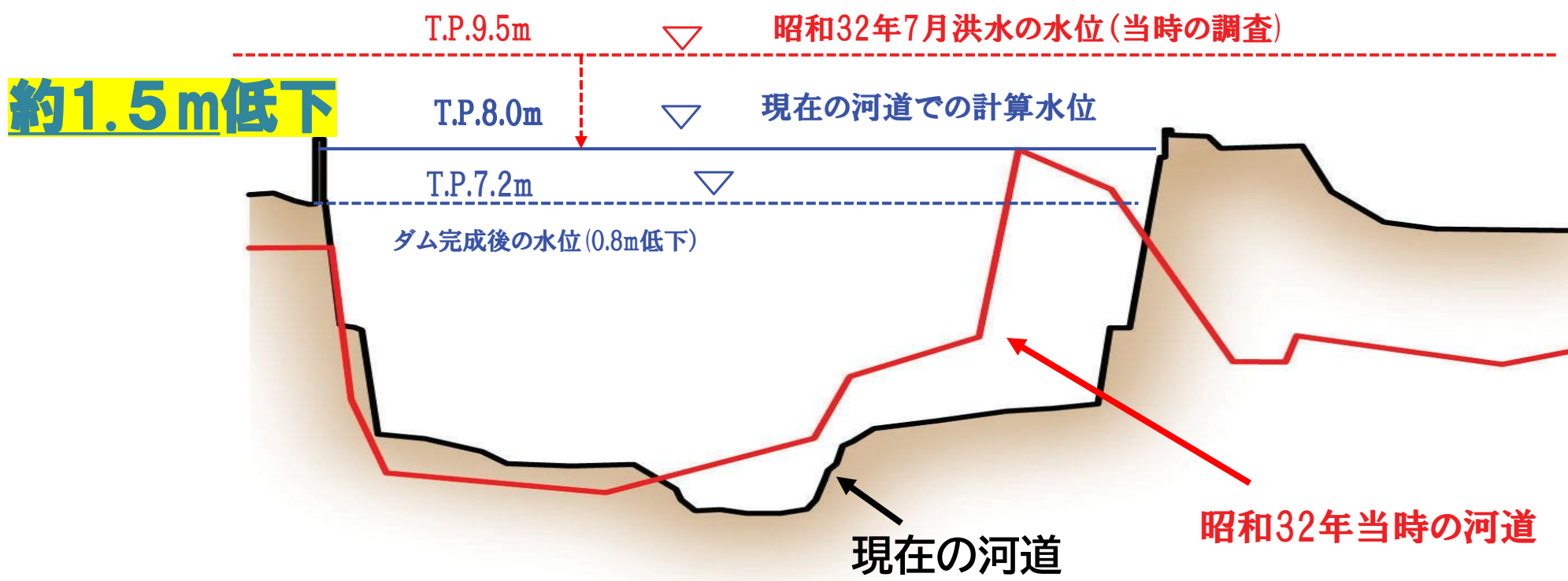
○高城橋水位断面図
