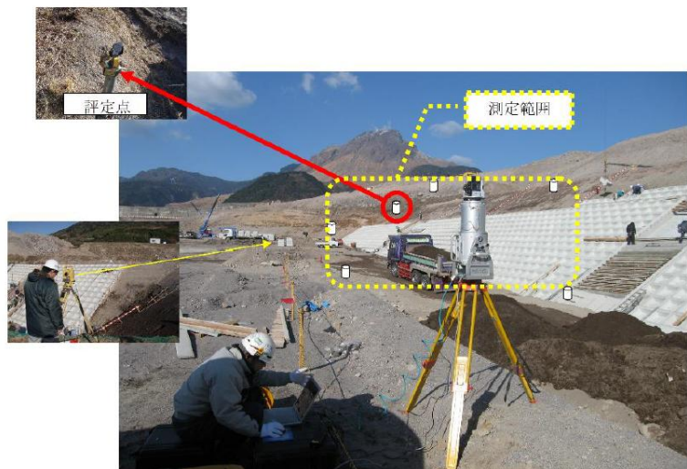
LSと標定点の配置(例)
