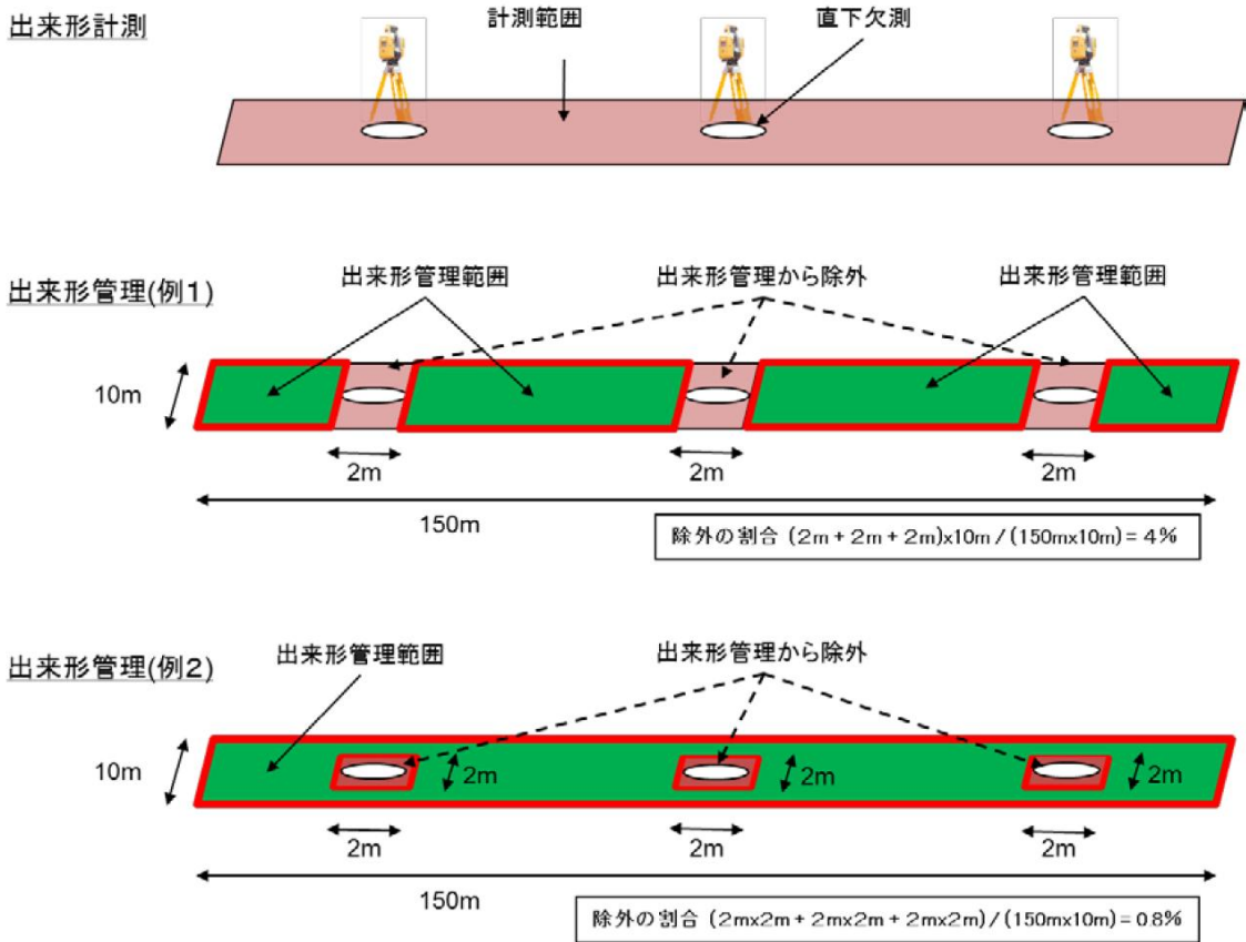
TLS直下の欠測の除外例
