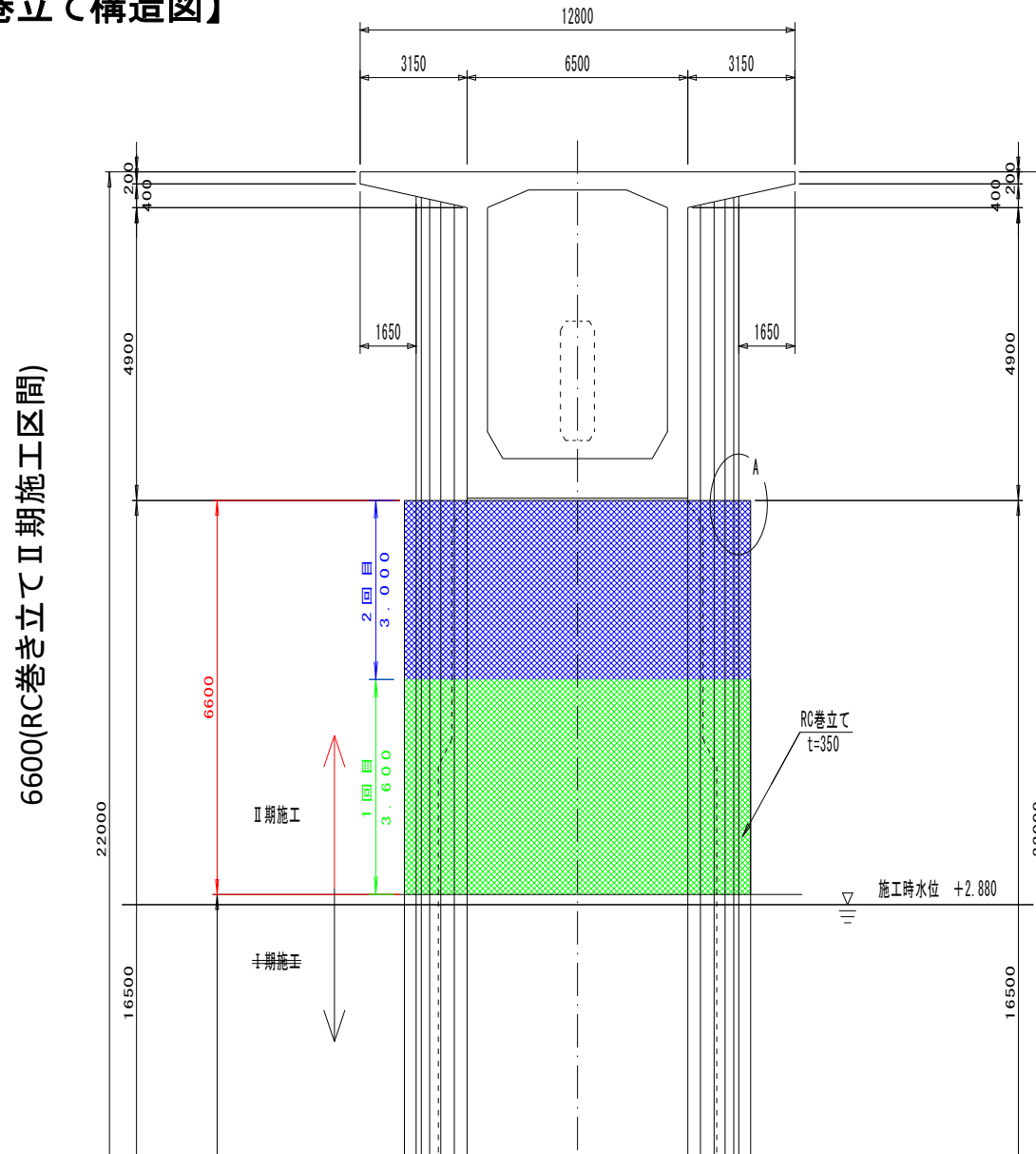
【巻立て構造図】
