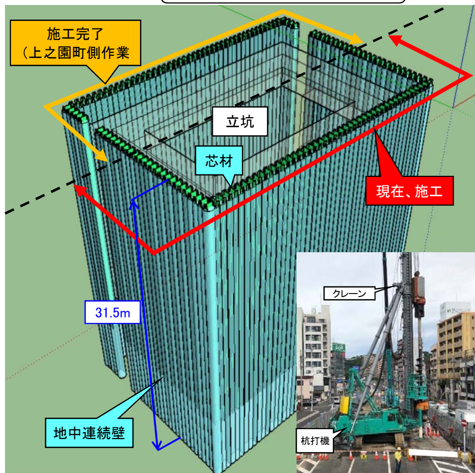
地中連続壁イメージ図(3D)
