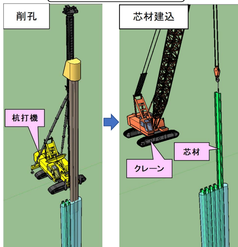
地中連続壁施工手順(3D)
