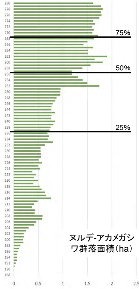
主要な群落の標高別植生面積
