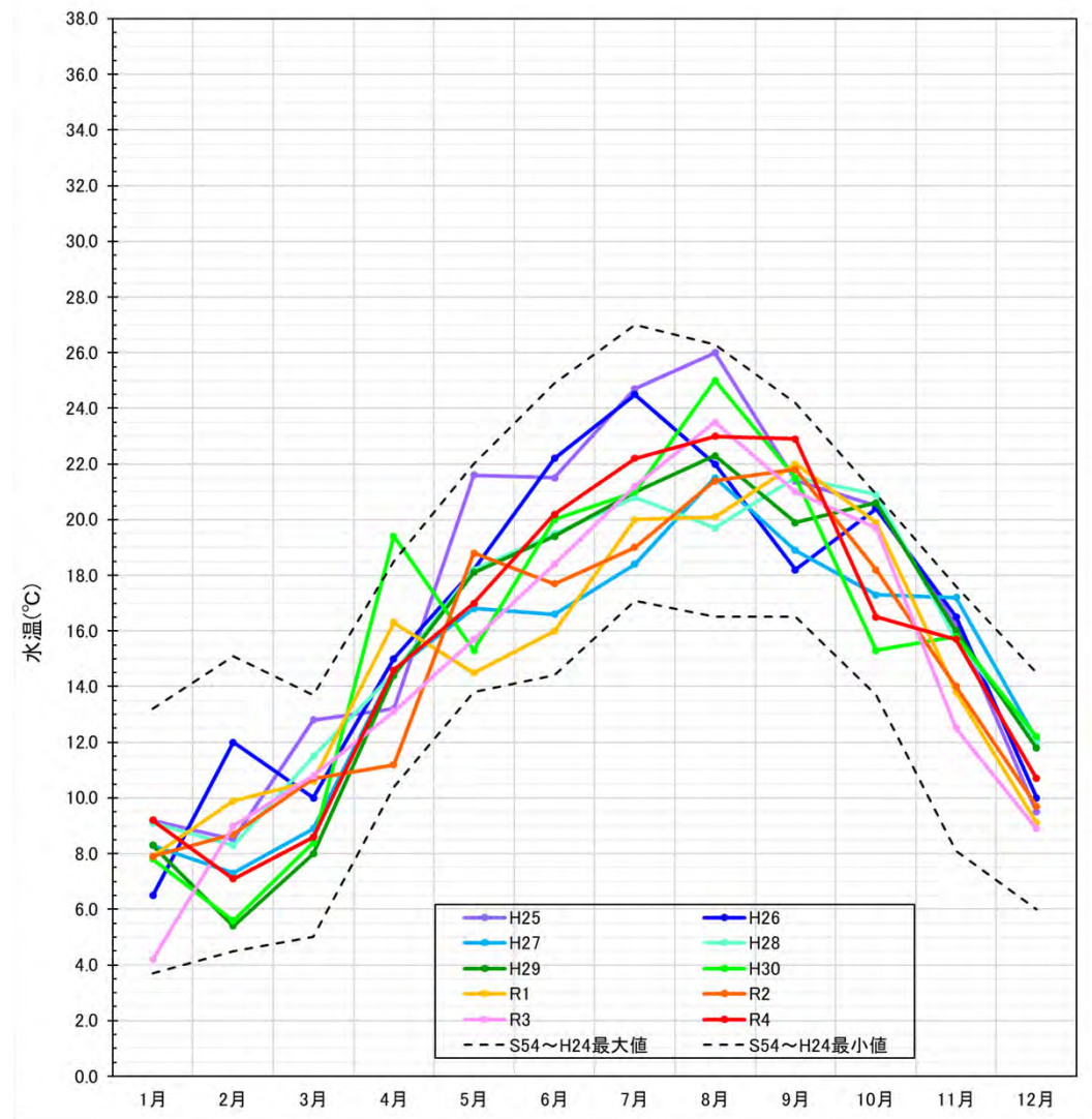
川辺川(四浦(ダム地点下流))における「水温」の各年の経月変化(S54~R4)
