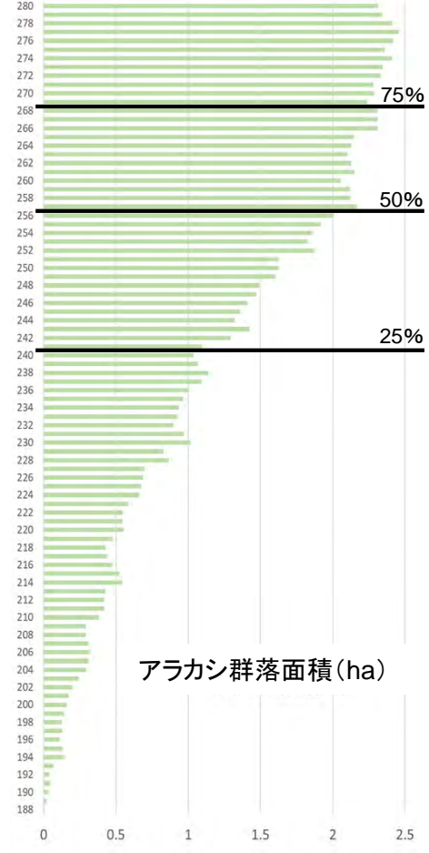
主要な群落の標高別植生面積
