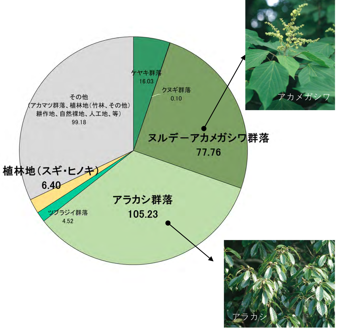
ダム洪水調節地内の植生内訳
