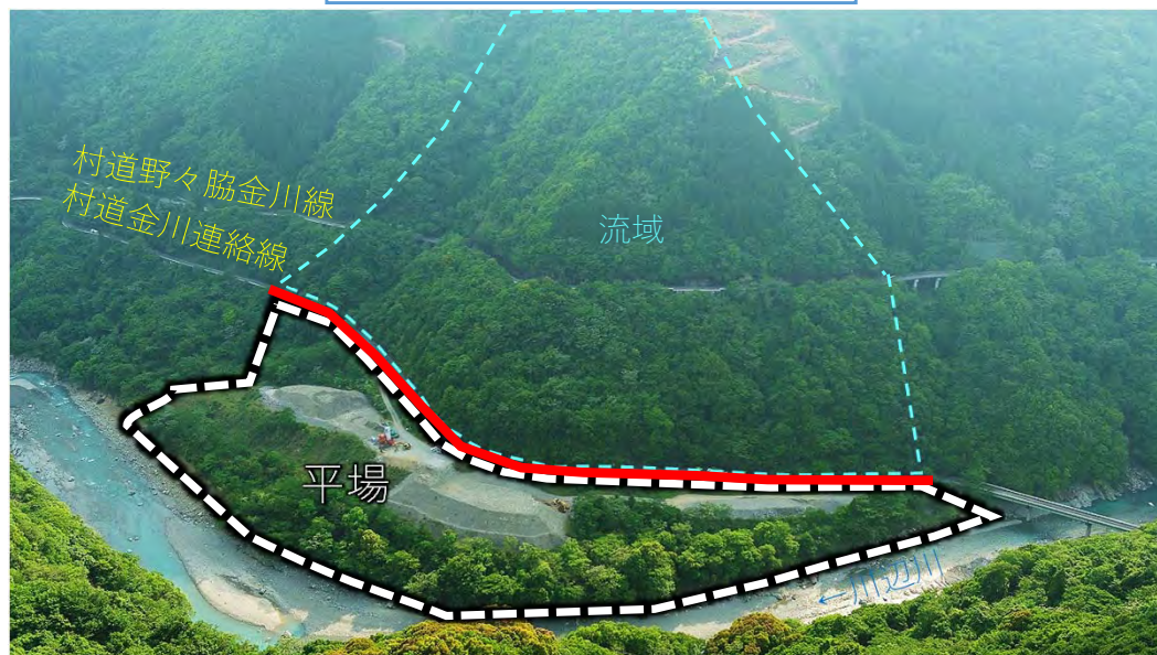
排水路対策イメージ図
