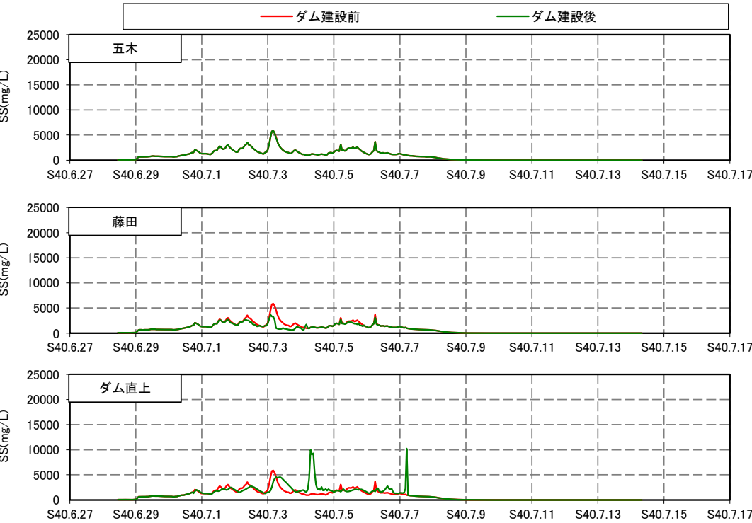
■昭和40年7月洪水 土砂による水の濁り
