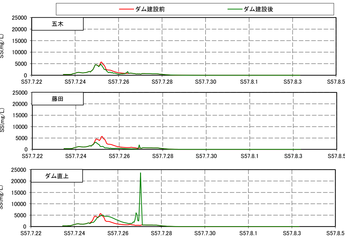
■昭和57年7月洪水 土砂による水の濁り
