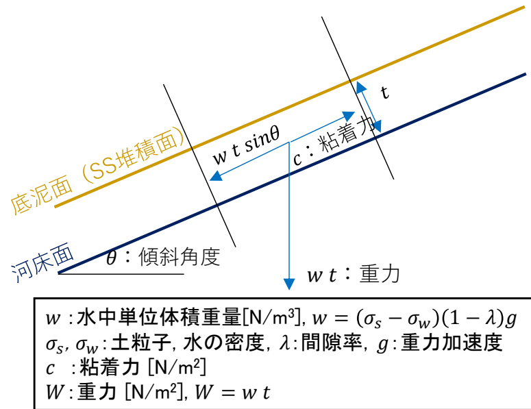
図 限界安息角における底泥層にかかる重力と粘着力の力のつり合い
