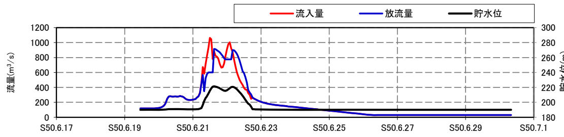
■昭和50年6月洪水 流入・放流・貯水位
