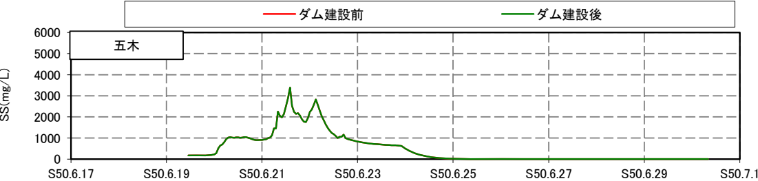
■昭和50年6月洪水 土砂による水の濁り
