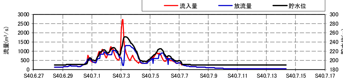
■昭和40年7月洪水 流入・放流・貯水位
