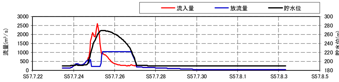
■昭和57年7月洪水 流入・放流・貯水位
