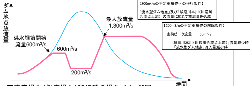
不定率操作(鍋底操作)移行時の操作イメージ図
