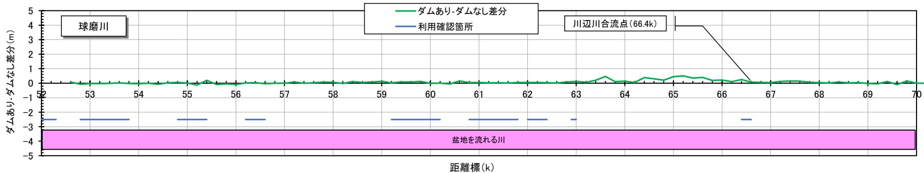
ダムあり(ダム建設後)とダムなし(ダム建設前)の場合の球磨川の河床高の変化と河床高の差分(10年後)
