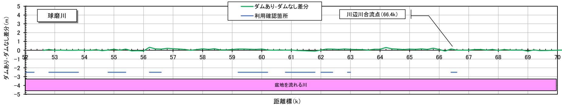
ダムあり(ダム建設後)とダムなし(ダム建設前)の場合の球磨川の河床高の変化と河床高の差分(100年後)
