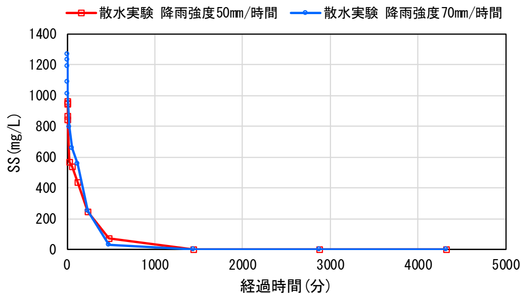
図 沈降試験結果
