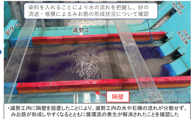
減勢工内に隔壁を設置した場合の実験の様子
