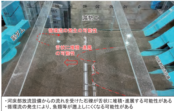
減勢工内の幅が広い場合の実験の様子
