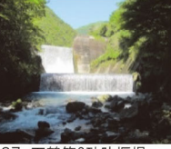
87. 下鶴第3砂防堰堤 完成: 平成6年7月 堤高: 14.50m
