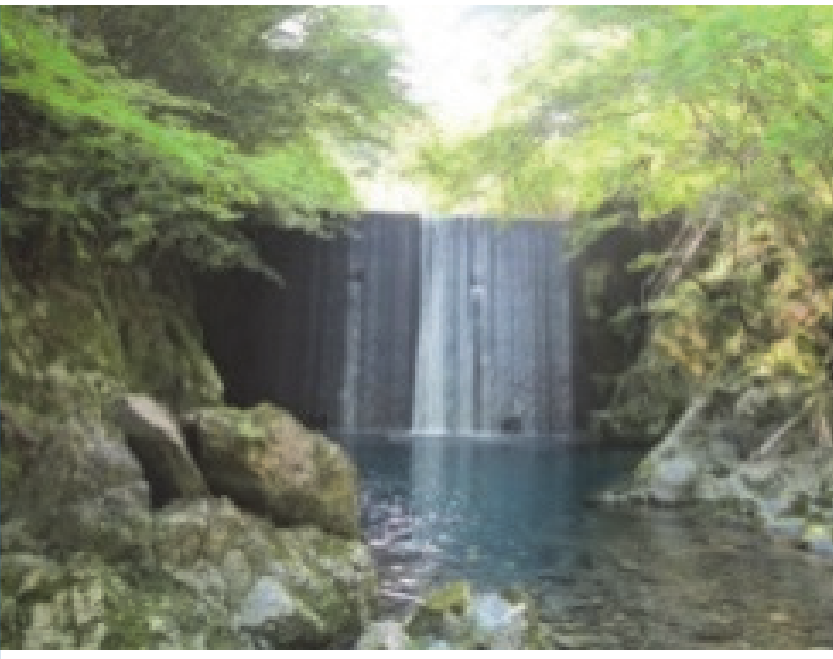
1. 飯干川第2砂防堰堤 完成：昭和43年2月 堤高：9.50m
