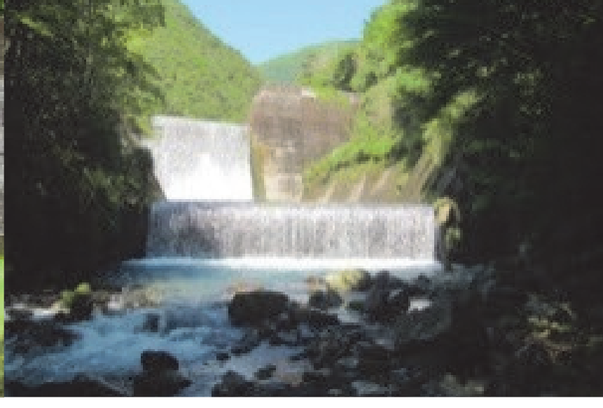
87. 下鶴第3砂防堰堤 完成: 平成6年7月 堤高: 14.50m
