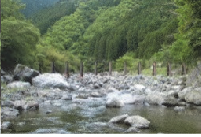
93. 小川砂防堰堤 完成: 平成8年3月 堤高: 8.00m
