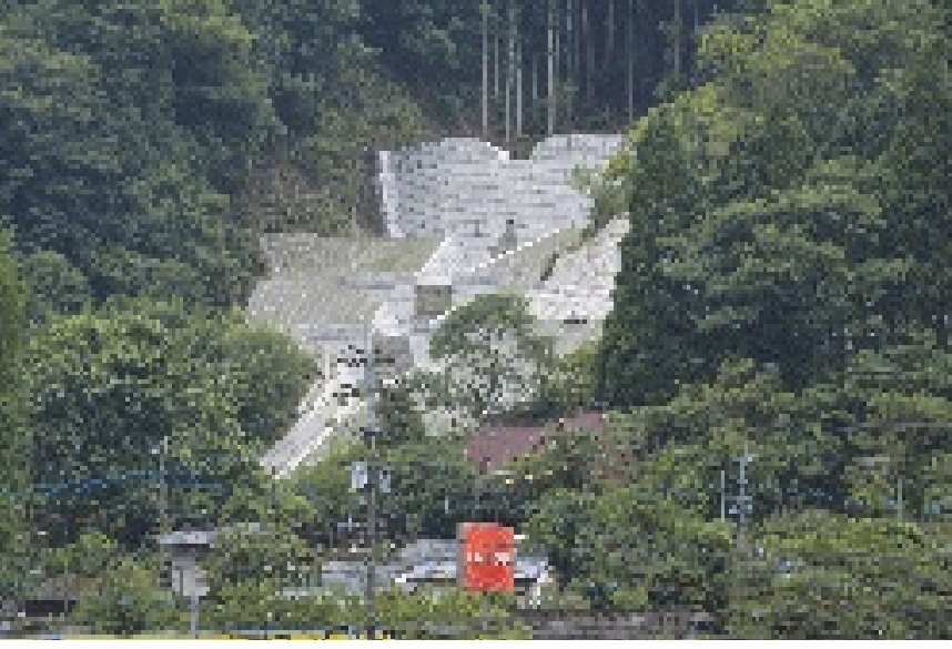
119. 宮園砂防堰堤 完成: 平成29年6月 堤高: 11.00m
