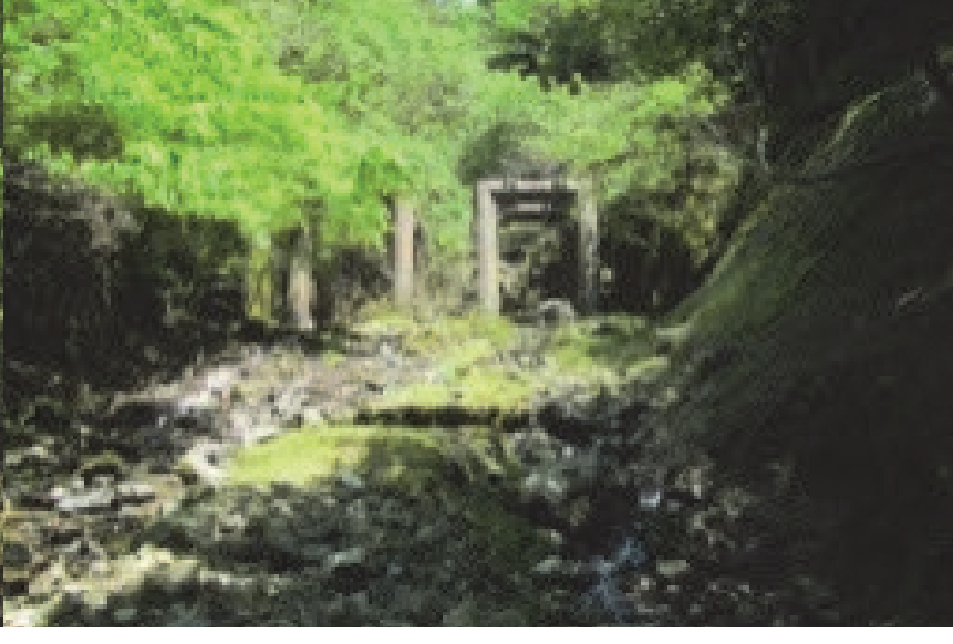
85. 内谷第5砂防堰堤 完成: 平成6年3月 堤高: 7.00m
