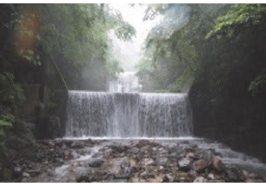
63. 元井谷川砂防堰堤 完成: 昭和60年6月 堤高: 15.00m
