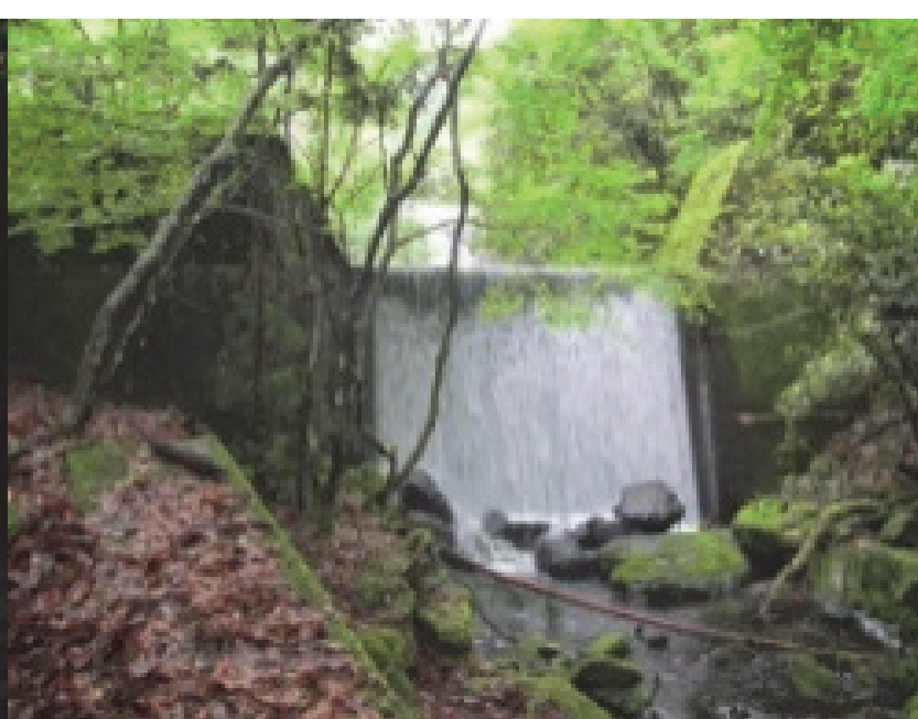
59. 大谷谷川第2砂防堰堤 完成：昭和58年1月 堤高：14.00m
