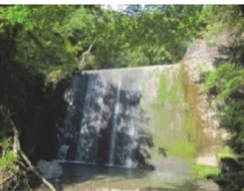
50. 白岩戸砂防堰堤 完成：昭和54年3月 堤高：10.00m
