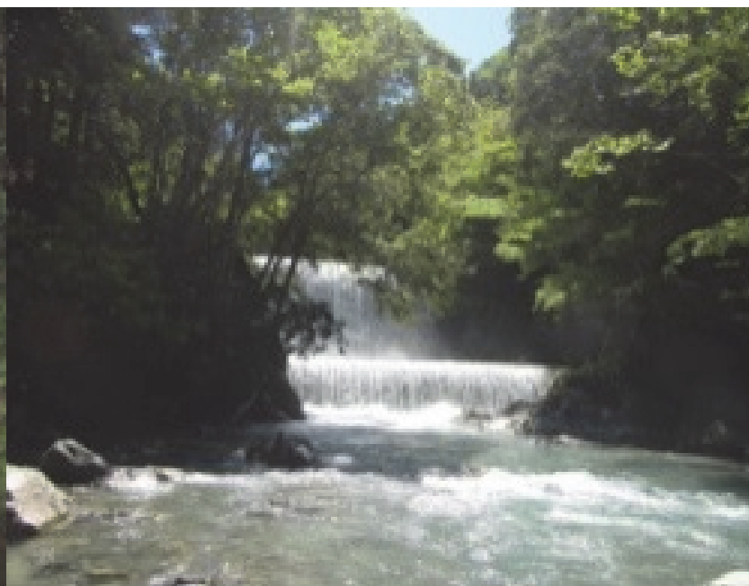
45. 空舎第3砂防堰堤 完成：昭和53年1月 堤高：14.50m
