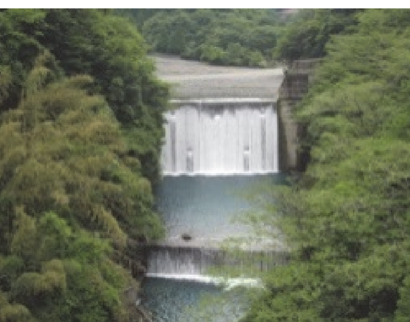
56. 朴木砂防堰堤 完成：昭和55年3月 堤高：25.00m
