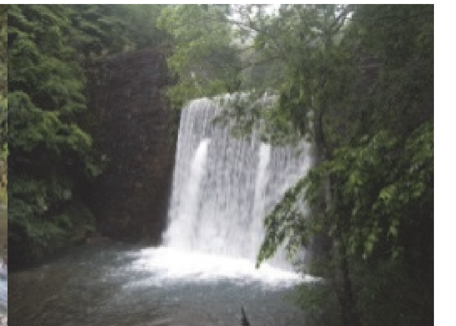
47. 山口谷川第2砂防堰堤 完成：昭和53年3月 堤高：16.50m
