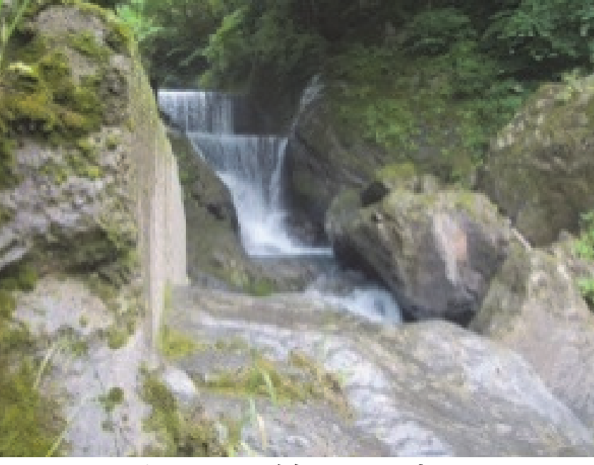
6. 西内谷川第2砂防堰堤 完成：昭和43年11月 堤高：12.00m
