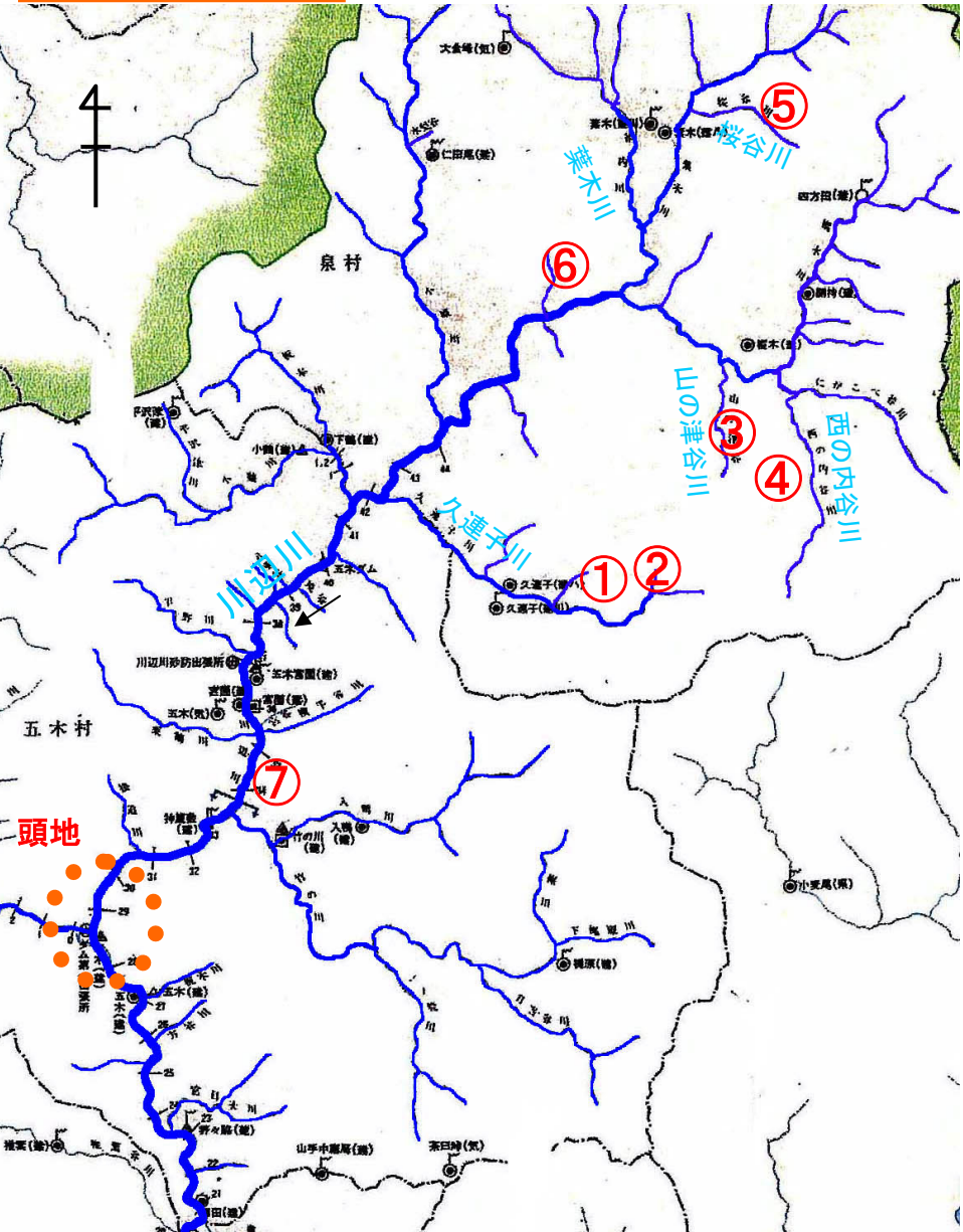
土砂崩壊位置図
