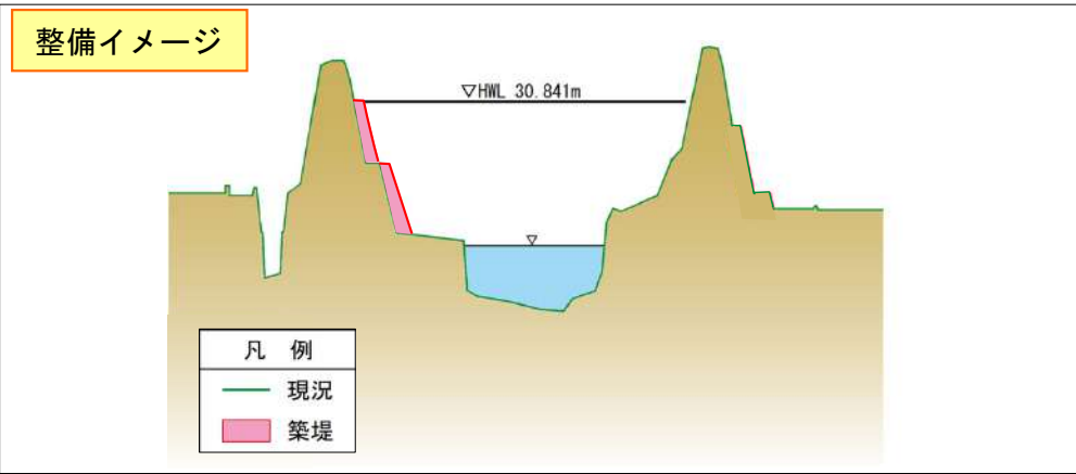
菊池川 42k000(横断図)
