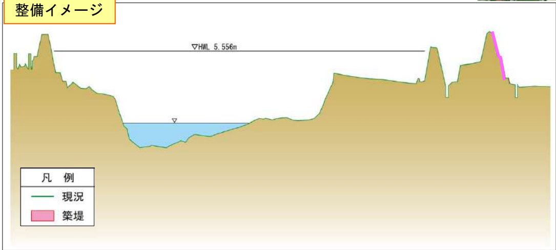
菊池川 3k000(横断図)
