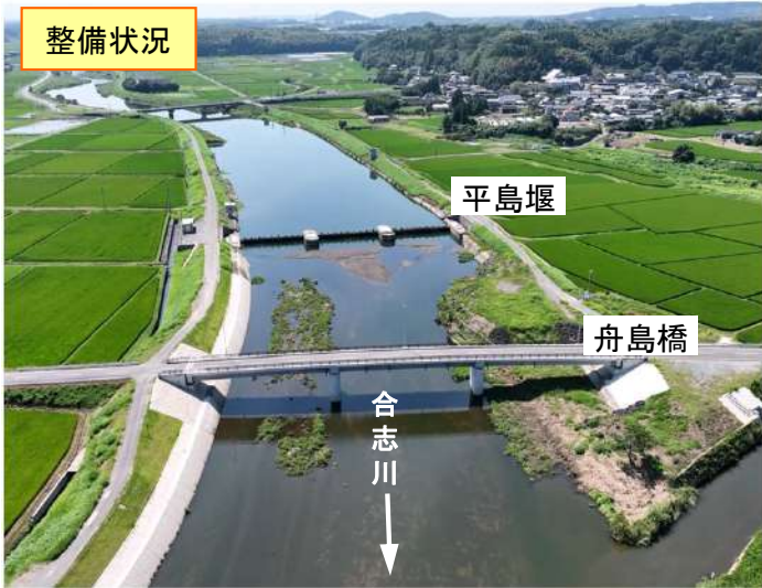
平島堰改築・舟島橋架替(整備後)
