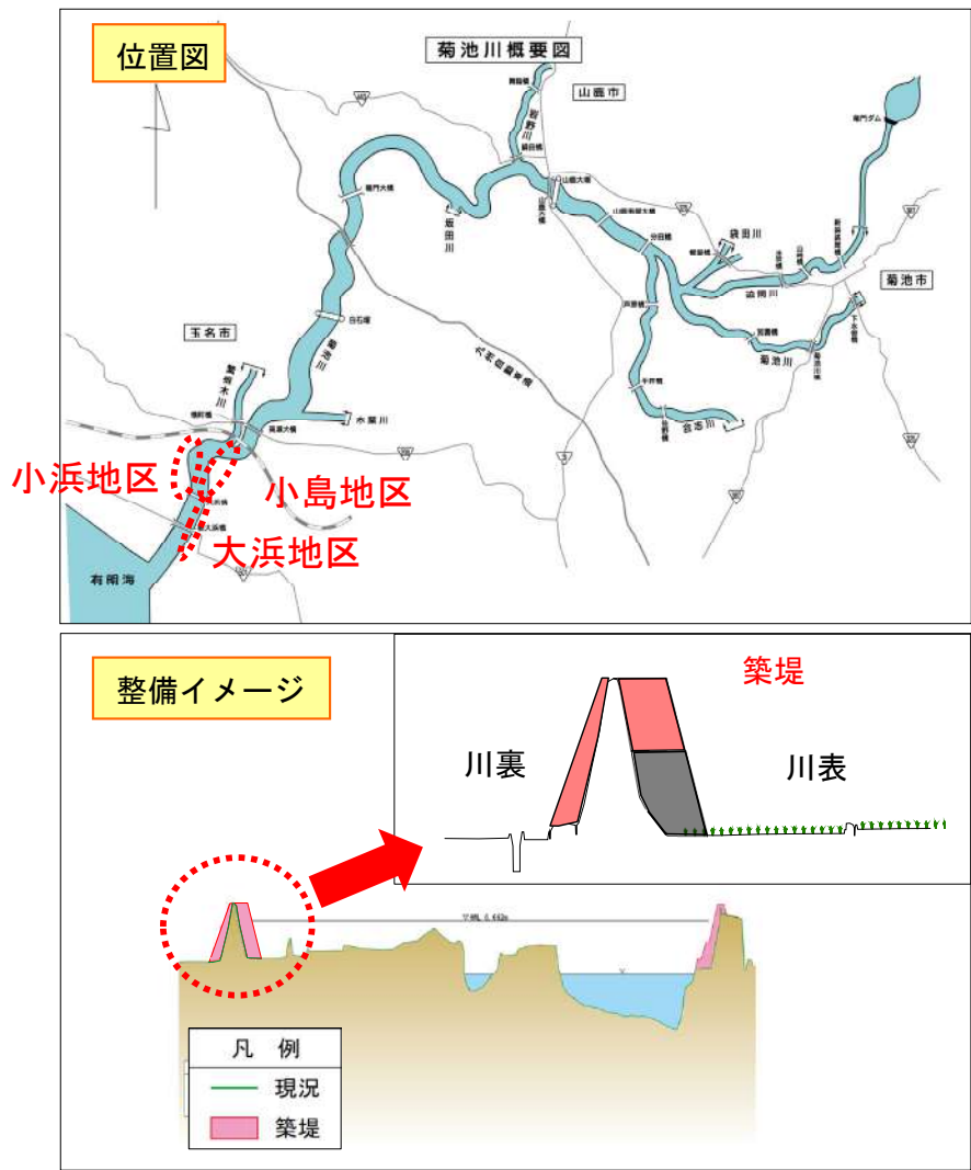
菊池川 4k800(横断図)
