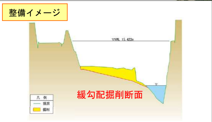
菊池川 20k200(横断面図)
