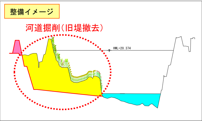
菊池川 28k600(横断図)
