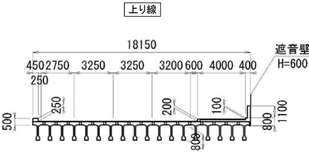
標準断面図
