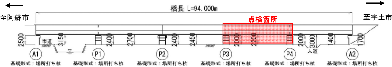
側面図
