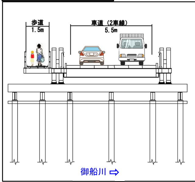
応急組立橋断面図
