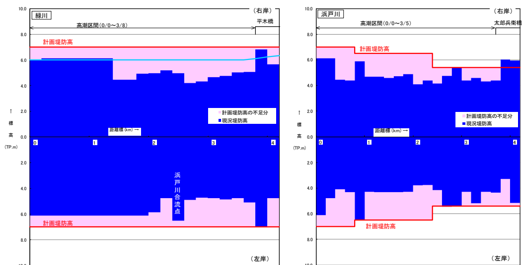
図 2.1-5 緑川・浜戸川高潮堤防高縦断面図 (令和5年(2023年)3月現在)
