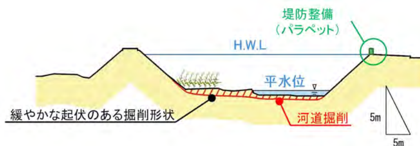
図 4.2-15 整備イメージ図（秋津川 2k800 付近）
