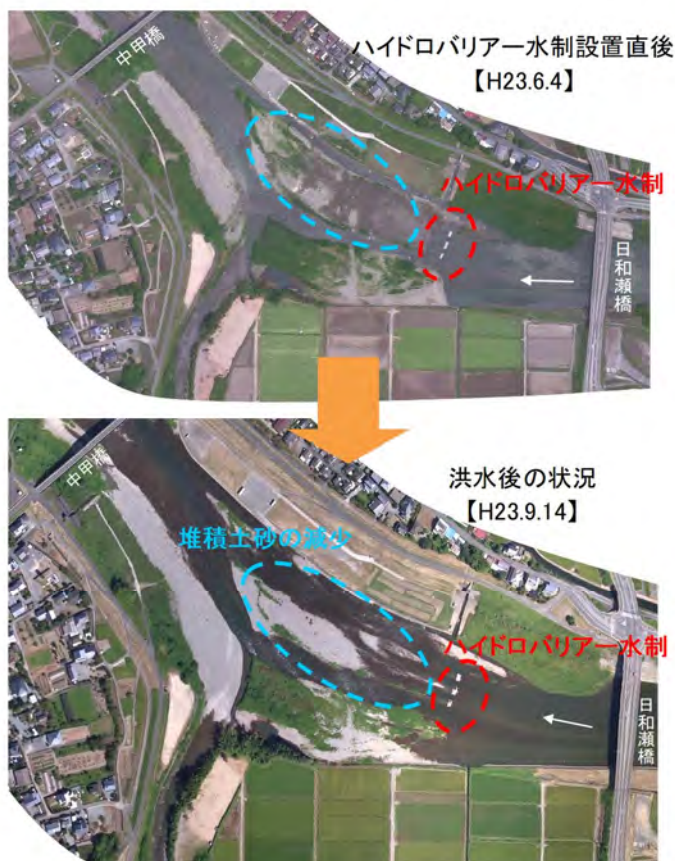
写真 4.3-14 土砂堆積部の河道管理
