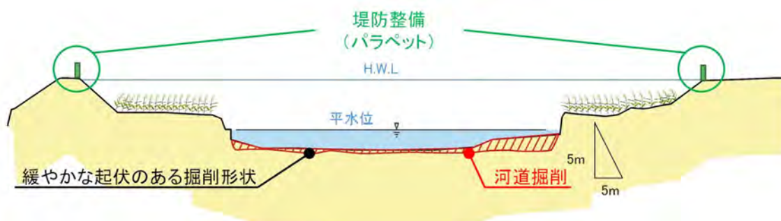
図 4.2-13 整備イメージ図（木山川 12k000 付近）
