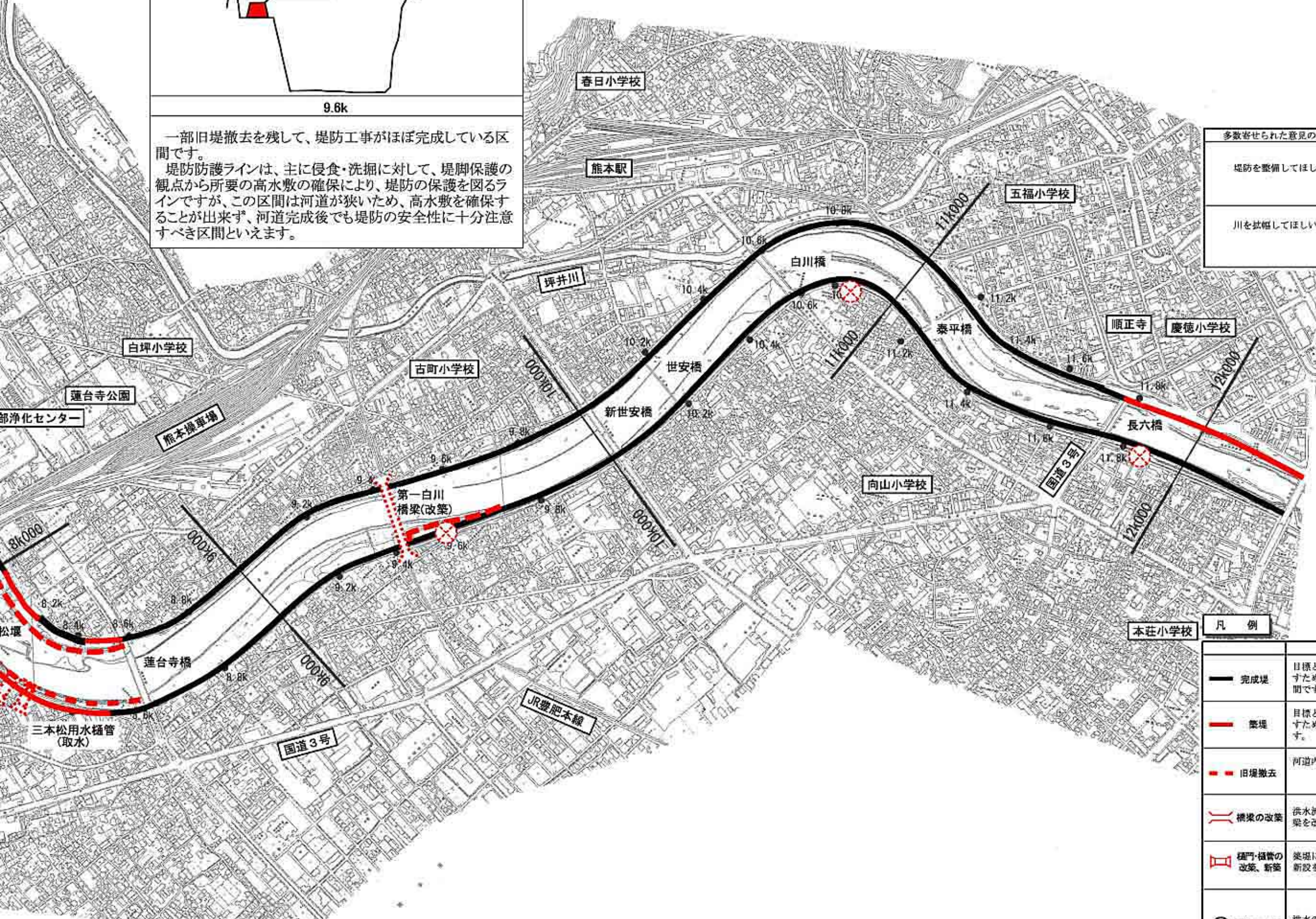
河川整備計画図(治水対策)
