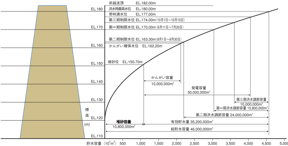
貯水池容量配分図
