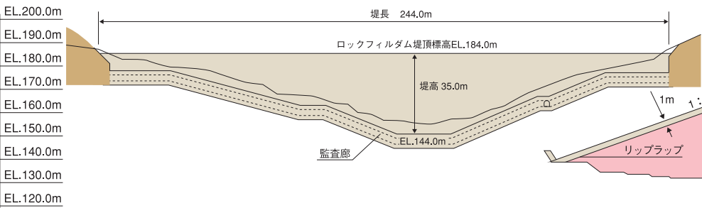
脇ダム(ロックフィルダム)上流面図
