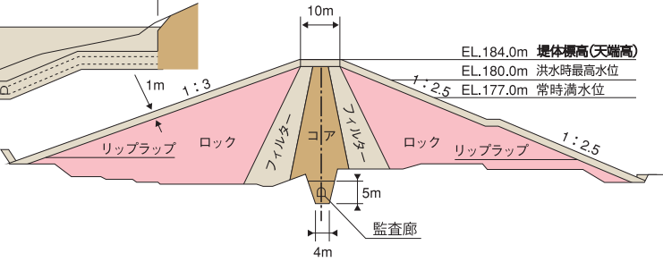
脇ダム標準断面図
