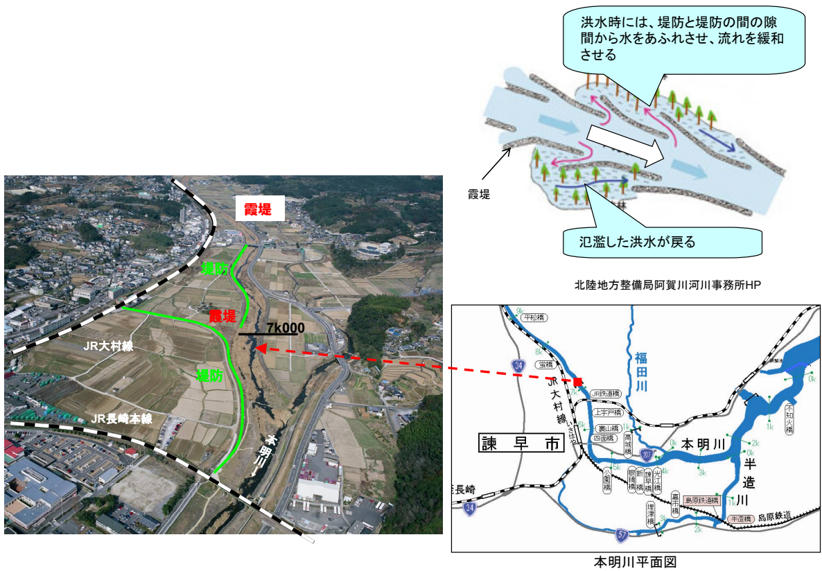
図 4.2-14 霞堤の存置のイメージ
