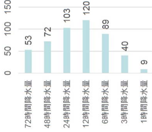
観測史上1位の更新地点数 (時間降水量別)
