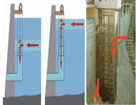
選択取水設備（事例）
