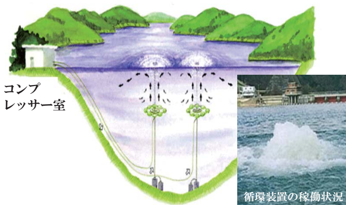
曝気循環設備（事例）
