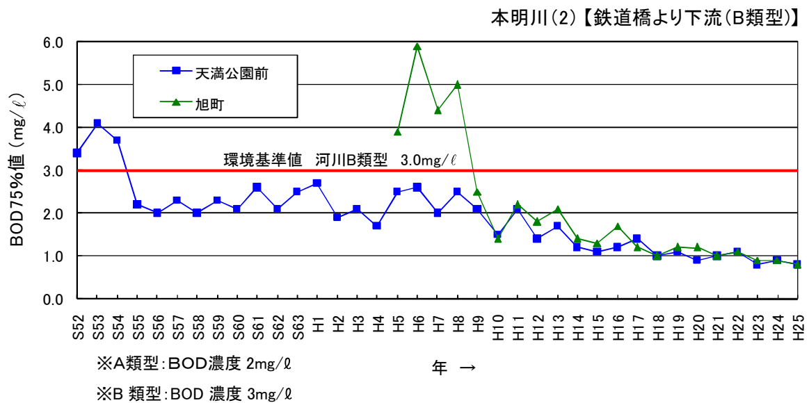
図2-3-3 本明川の各地点における水質(BOD75%値)の経年変化
