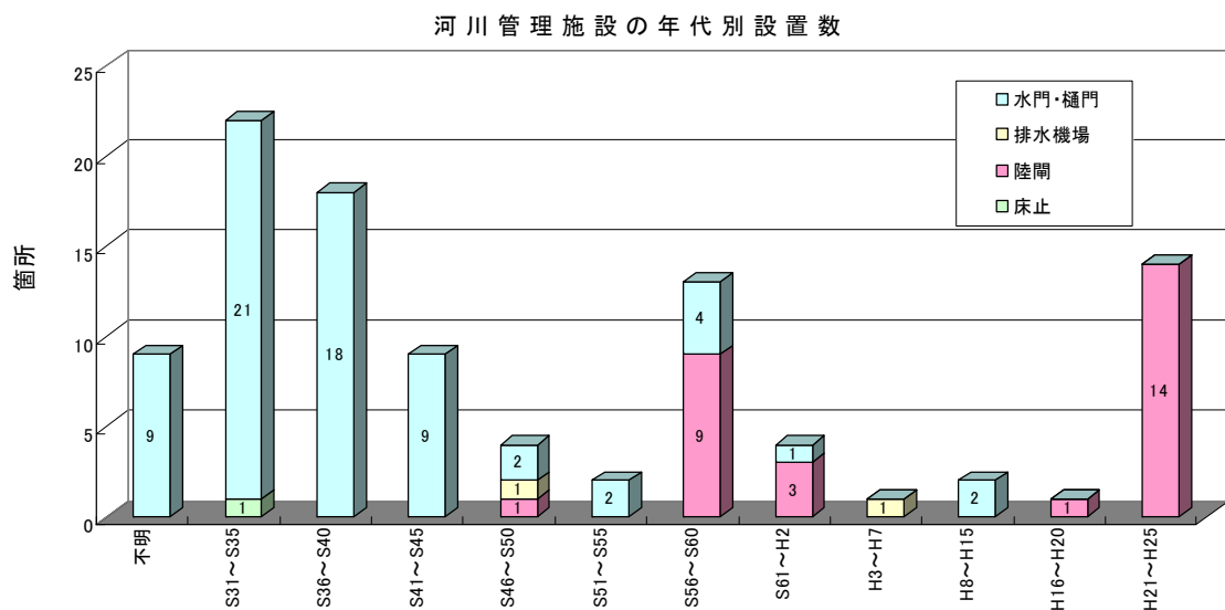
図2-1-3 河川管理施設の年代別設置数
