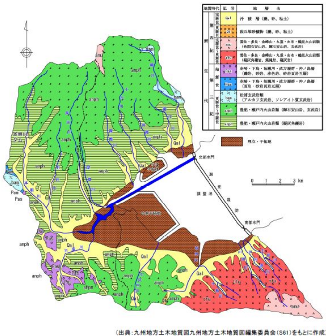
図1-1-3 本明川流域地質図
