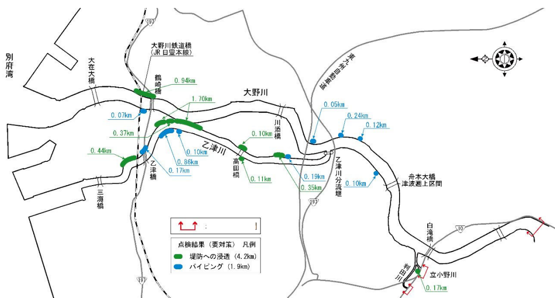
図 2.1.2 平成 24 年（2012 年）7 月の九州北部豪雨災害を踏まえた堤防の緊急点検結果 (出典：平成 24 年（2012 年）9 月 4 日発表、九州地方整備局)
