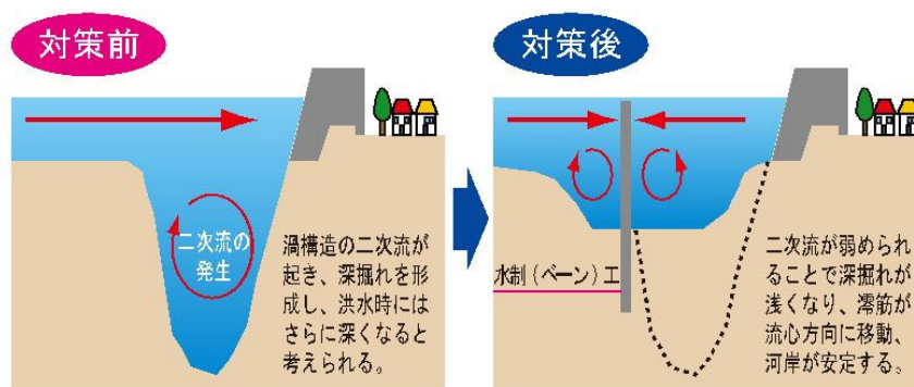
図 1.2.6 水制工の効果
