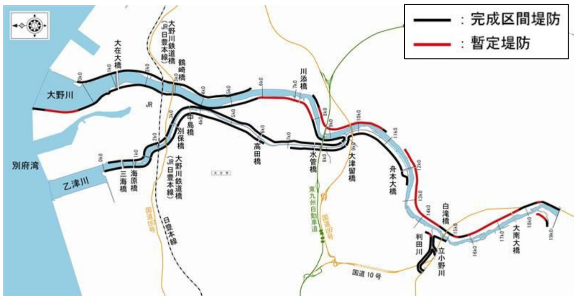
図 2.1.1 堤防整備状況（令和7年(2025年)3月末時点）
