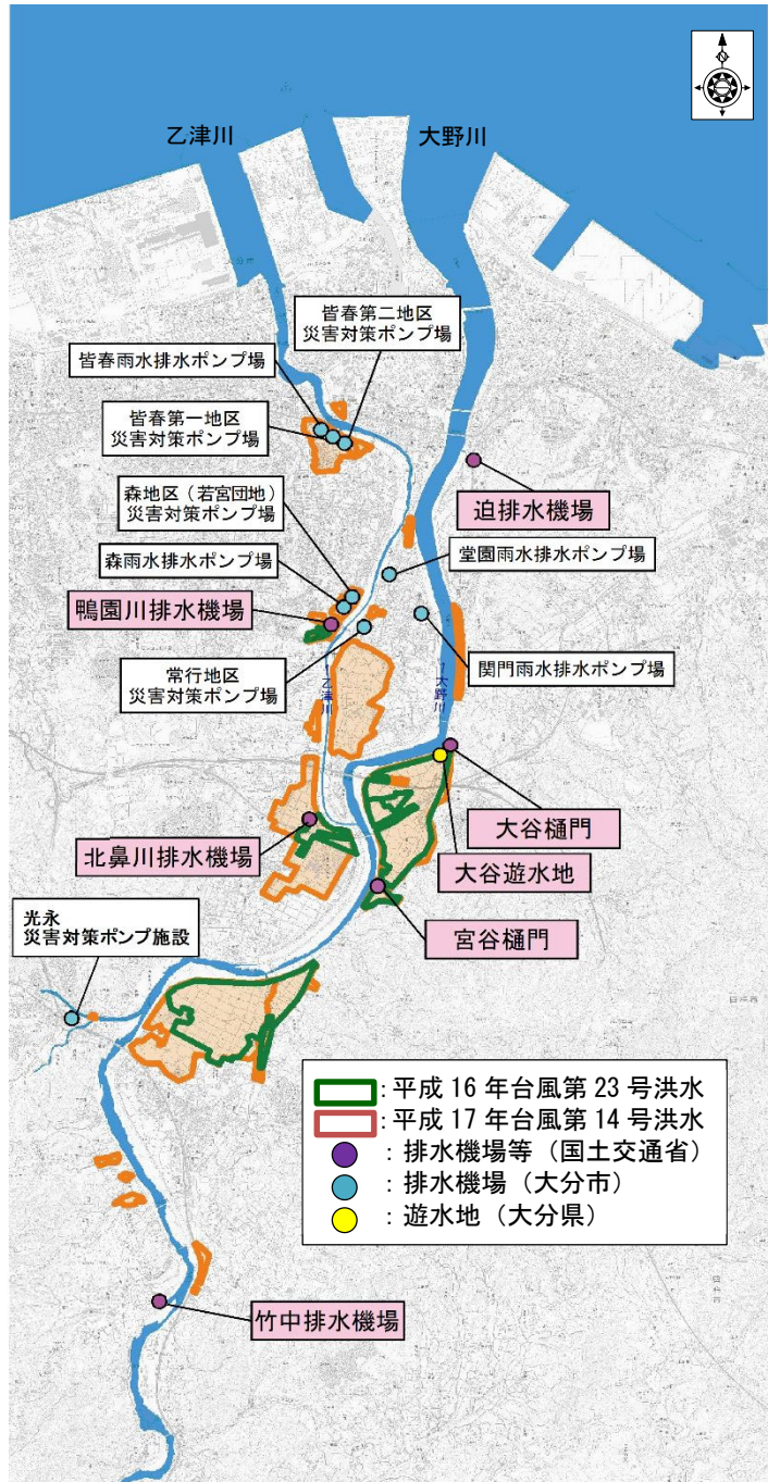
図 2.1.3 内水対策実施箇所位置図
