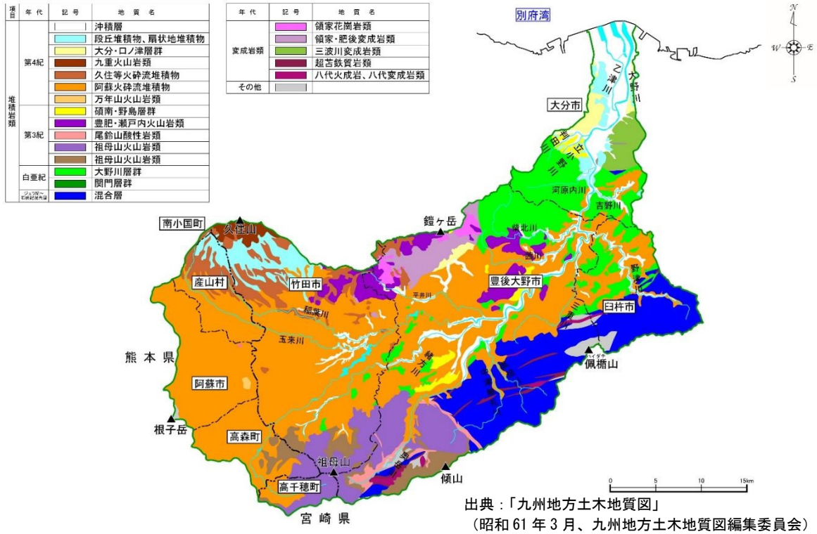
図 1.1.4 大野川流域地質図
