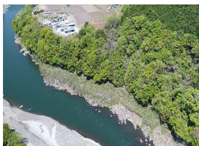
写真 2.3.7 アラカシ群落 (リバーパーク犬飼付近)
