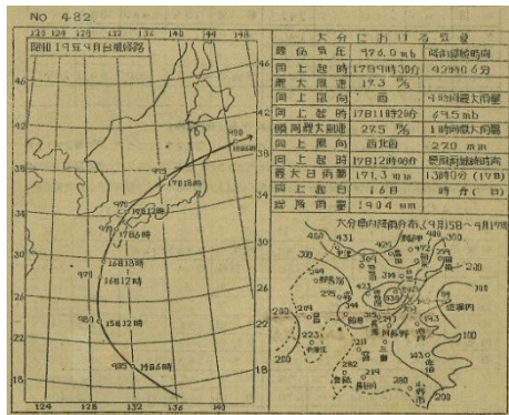
図 1.2.2 気象状況（昭和 18 年(1943 年)9 月洪水） （出典：大分県災害誌調査編(大分測候所)）
