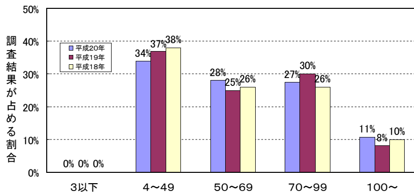
図-4 遠賀川水系における透視度調査結果のランク別割合
