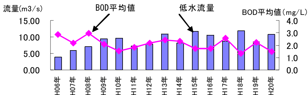
図－2－1 低水流量と水質の関係（日の出橋観測地点）
