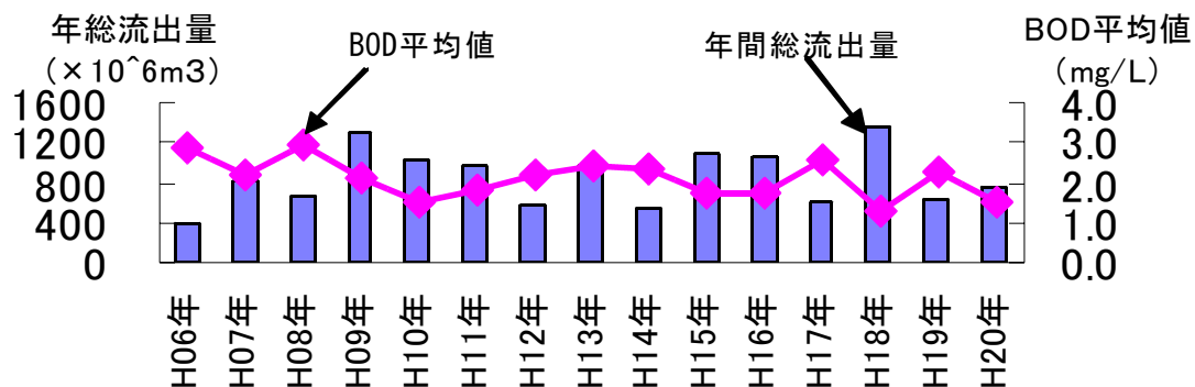
図－2－2 年間総流出量と水質の関係（日の出橋観測地点）
