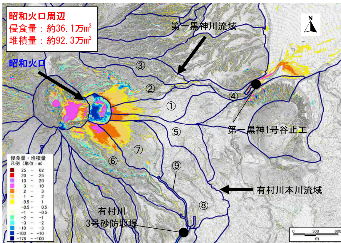
図4 昭和火口周辺侵食堆積図
