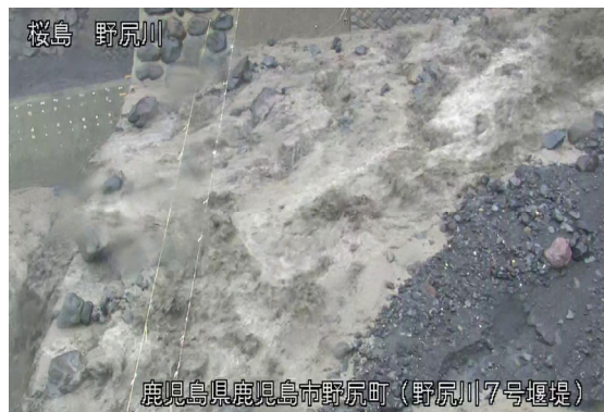
野尻川土石流の様子(5月6日)
