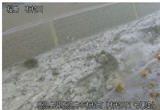
有村川土石流の様子(4月10日)
