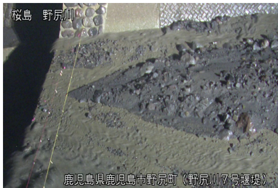
野尻川土石流の様子(5月9日)
