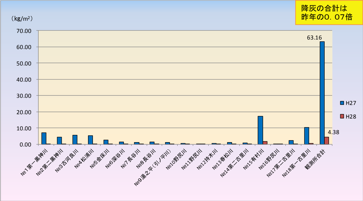
平成27年(1～2月)及び平成28年(1～2月)の降灰量比較
