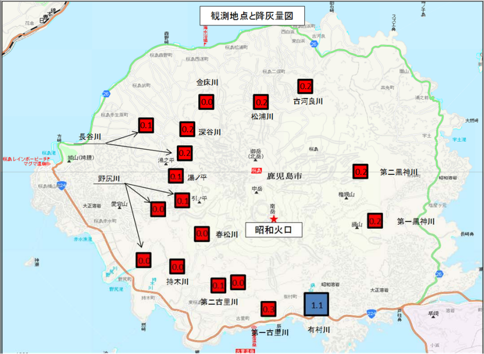
桜島の降灰観測結果(平成27年1月～12月)累計
