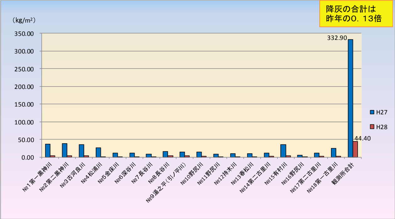
平成27年(1～8月)及び平成28年(1～8月)の降灰量比較
