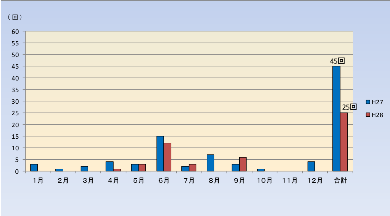
平成27年及び平成28年(1～9月)の土石流発生回数比較
