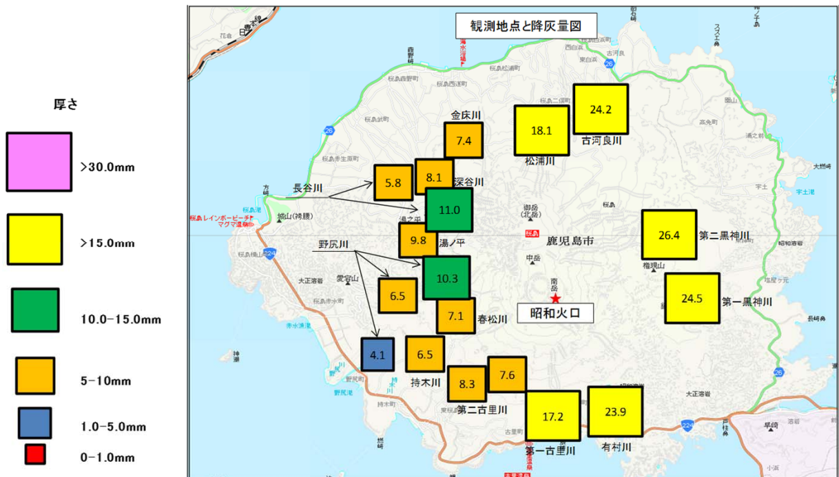
桜島の降灰観測結果(平成27年1月～12月)累計
