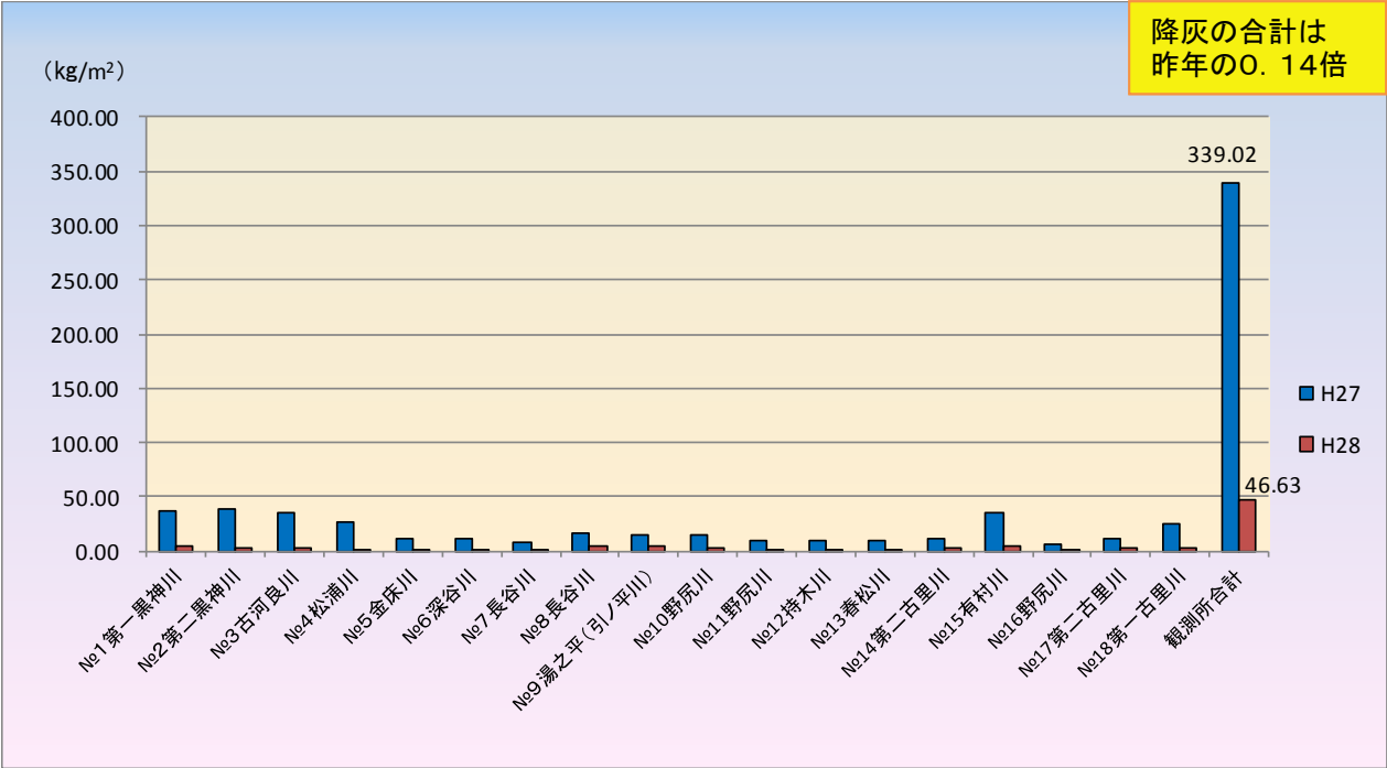
平成27年(1～10月)及び平成28年(1～10月)の降灰量比較
