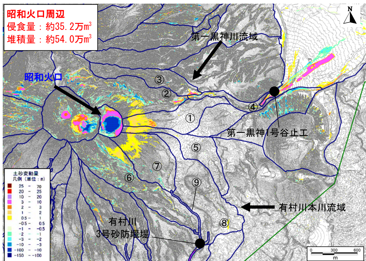
図4 昭和火口周辺侵食堆積図（平成27年11月～平成28年10月）
