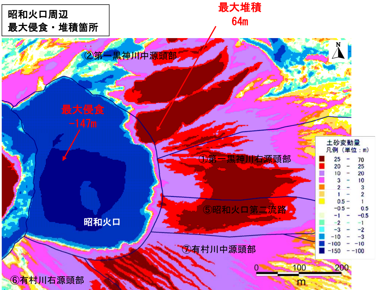
参考図6 昭和火口周辺最大侵食・堆積状況図（平成18年11月～平成28年10月）
