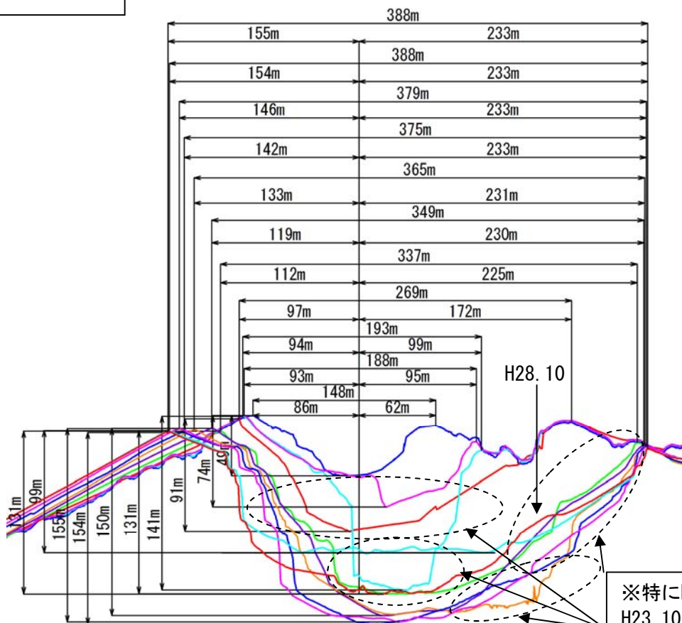
参考図5 昭和火口横断面拡大
