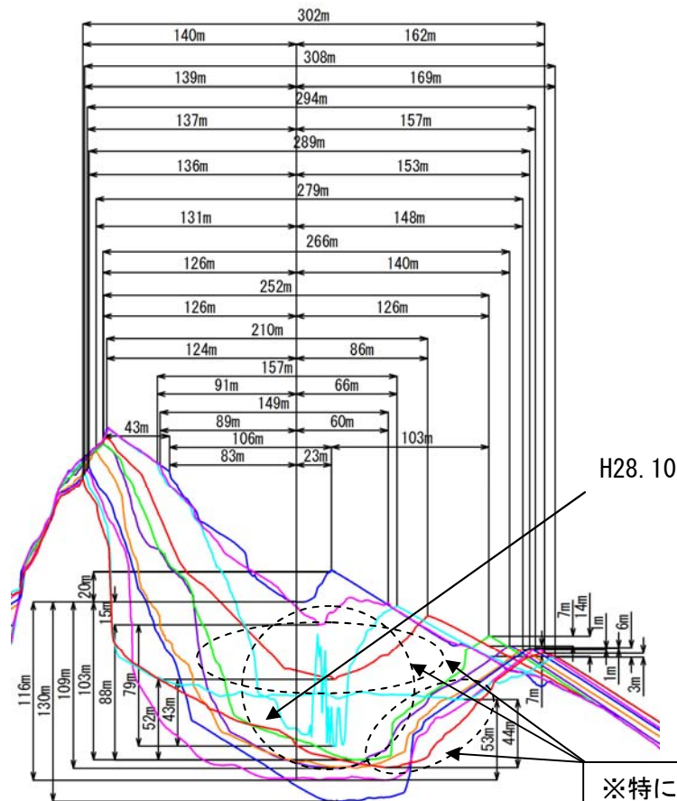
参考図4 昭和火口縦断面拡大
