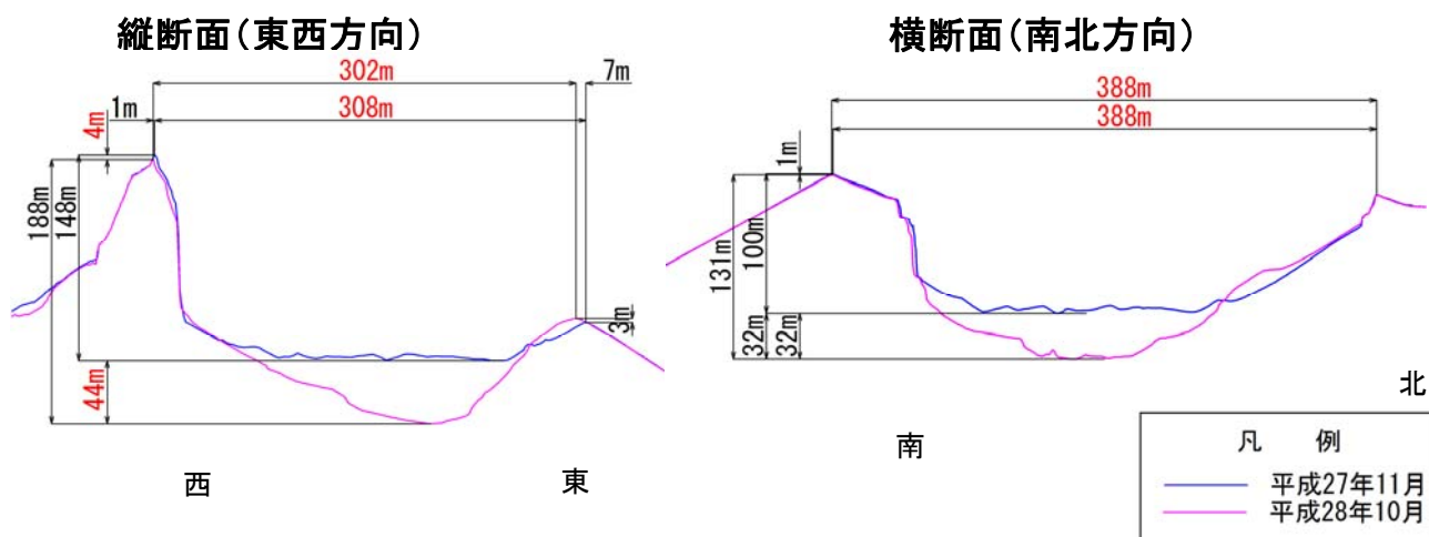
図2 昭和火口形状の経年変化（平成27年11月～平成28年10月）
