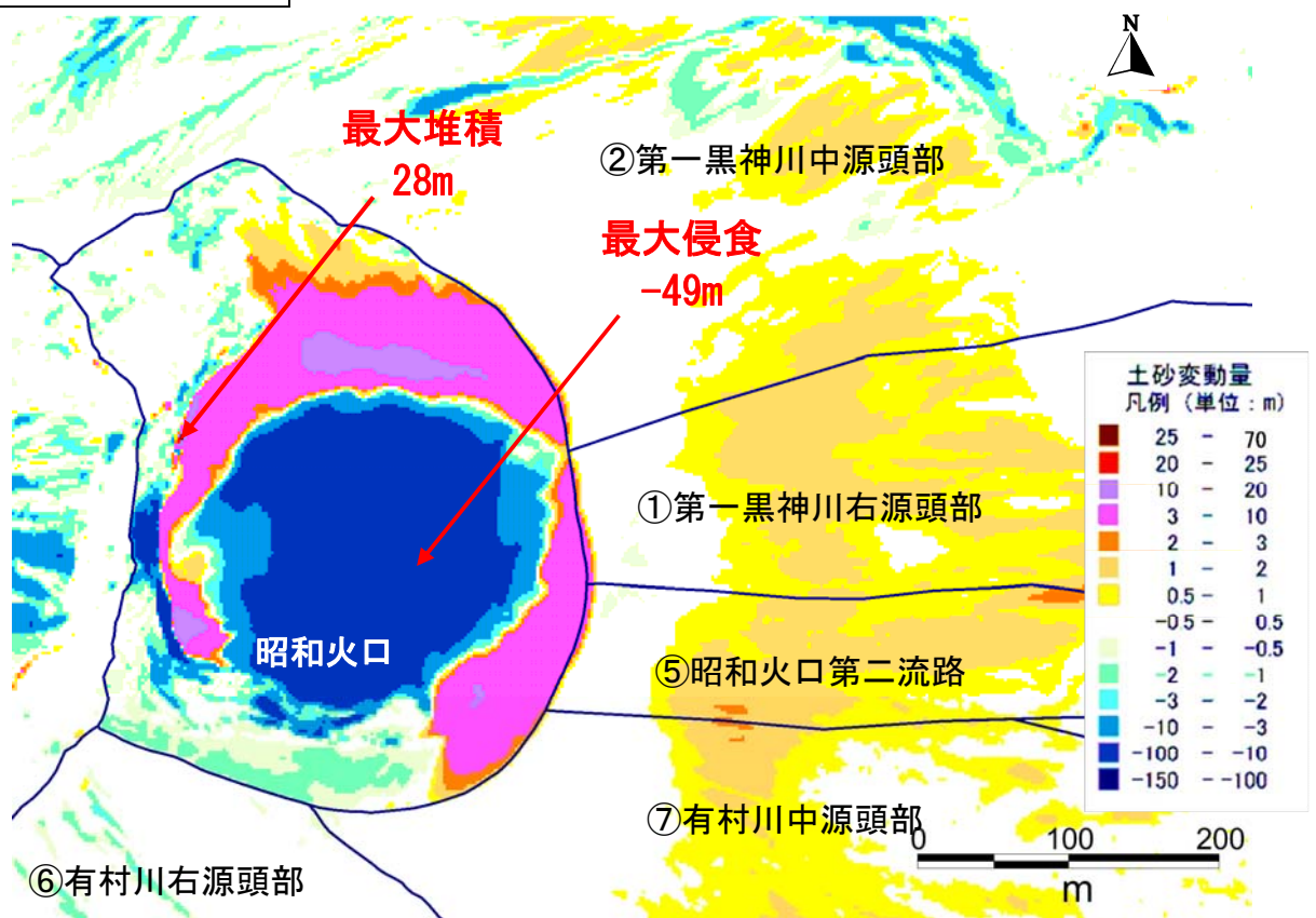
図3 昭如火口周辺最大侵食・堆積状況図 (平成27年11月～平成28年10月)
