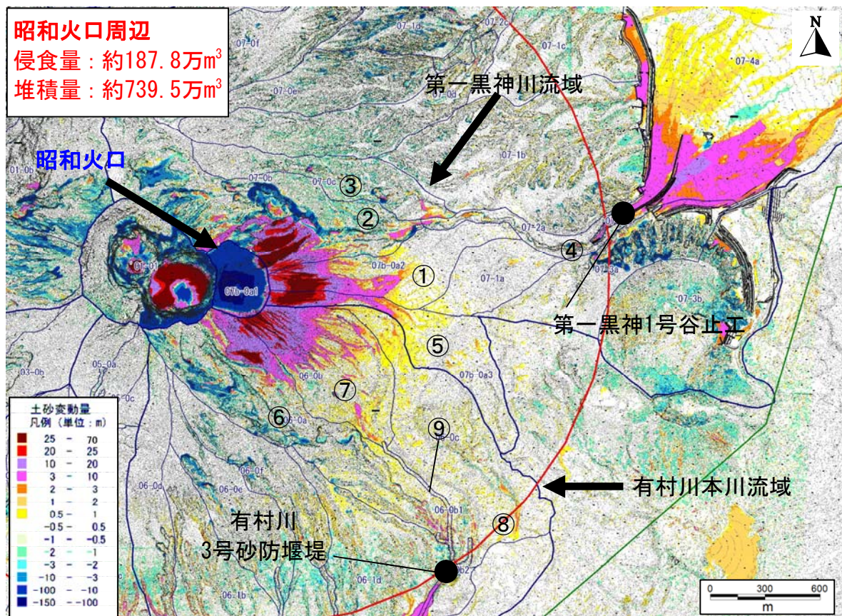
参考図7 昭和火口周辺侵食堆積図（平成18年11月～平成28年10月）
