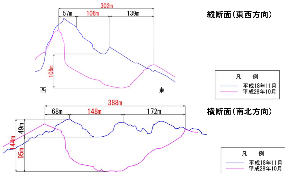
参考図2 昭和火口形状の経年変化（平成18年11月～平成28年10月）
