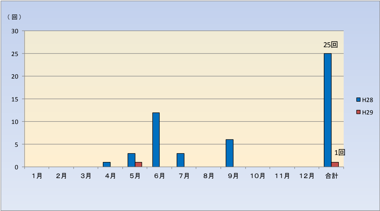
平成28年及び平成29年(1～4月)の土石流発生回数比較
