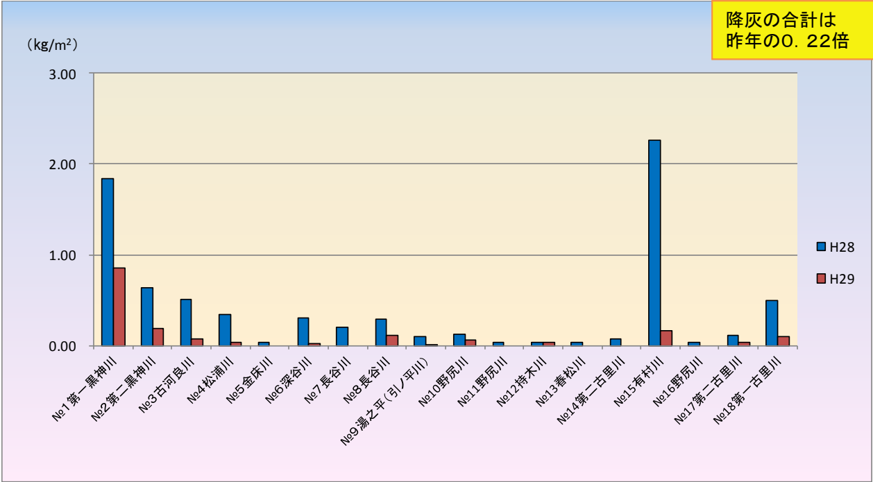
平成28年(1～3月)及び平成29年(1～3月)の降灰量比較
