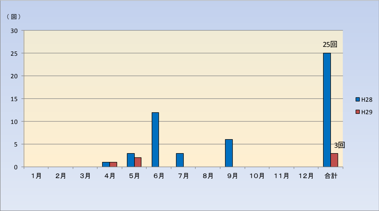
平成28年及び平成29年(1～5月)の土石流発生回数比較
