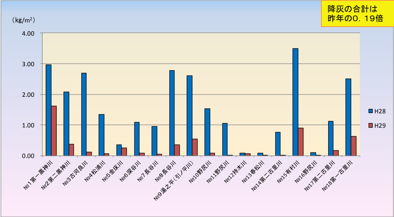
平成28年(1～4月)及び平成29年(1～4月)の降灰量比較
