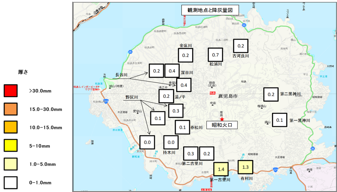
桜島の降灰観測結果(平成21年～平成29年)11月平均
