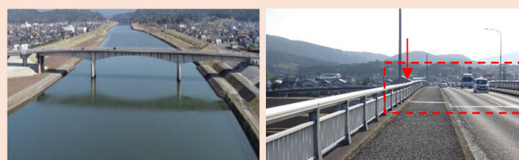
②天大橋（鹿児島県 薩摩川内市）：橋のつなぎ目の沈下等
