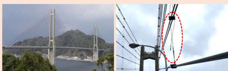
①呼子大橋（佐賀県 唐津市）：制振ワイヤーの損傷等
