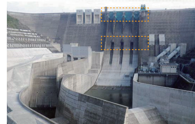
※ゲート設備構成 = ゲート本体 + 開閉装置 + 操作制御装置
