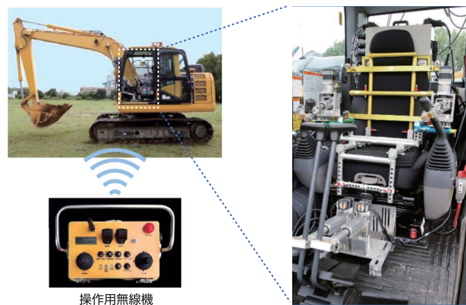
簡易遠隔操縦装置(ロボQS)
