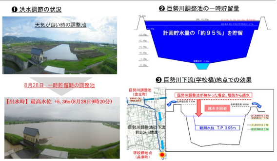
巨勢川調整池の効果（令和元年8月28日洪水）
