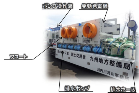
写真 4:排水ポンプ車
