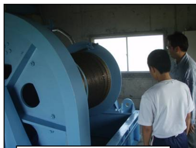
真幸堰ゲート巻上機
