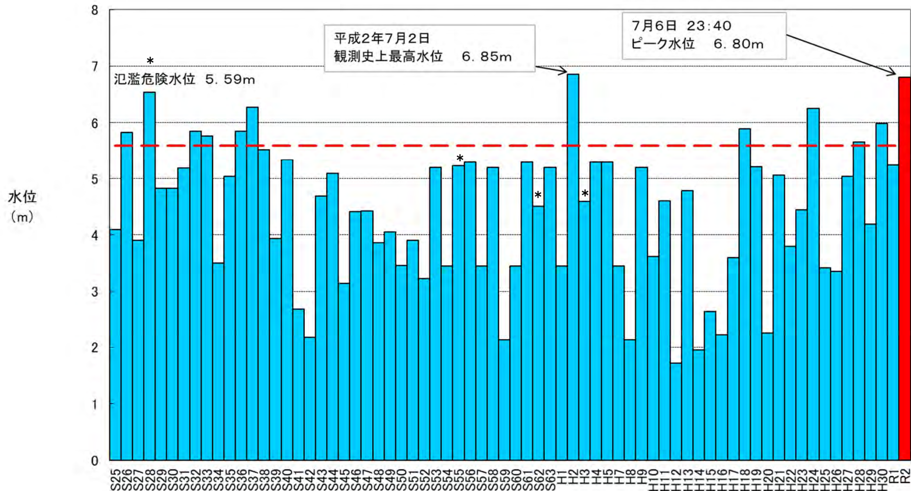
菊池川（玉名水位観測所の年最高水位比較図）
