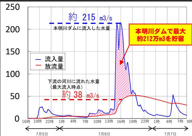
本明川ダムが完成した場合の状況
