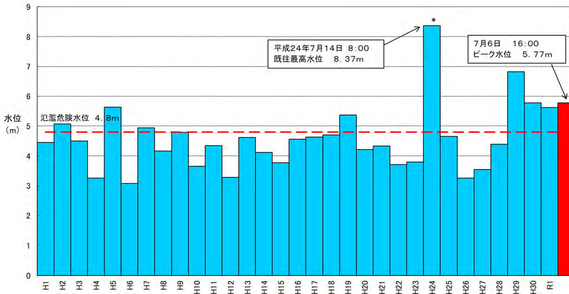
山国川（柿坂水位観測所の年最高水位比較図）
