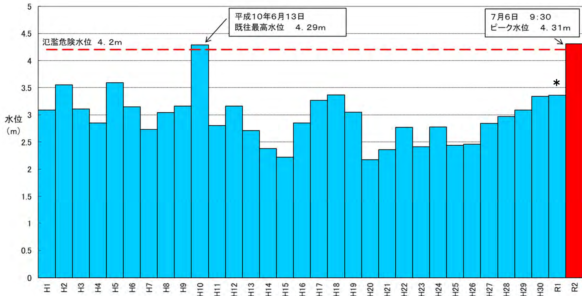
肝属川（王子橋水位観測所の年最高水位比較図）
