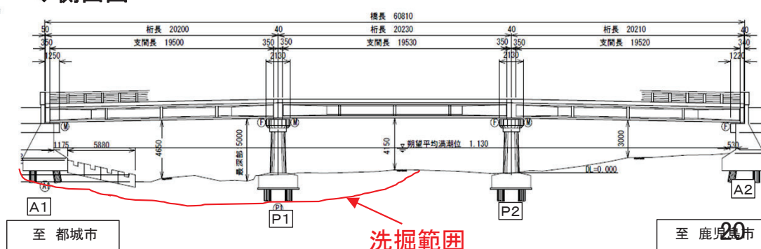
◆側面図
