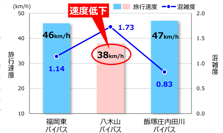
▲旅行速度の隣接区間比較
