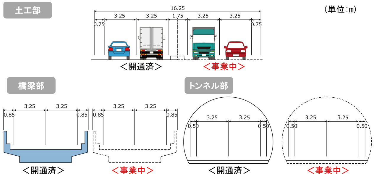
▲ 標準断面図
