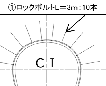
A-A断面
