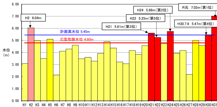
牛津川(妙見橋水位観測所)における年最高水位比較図
