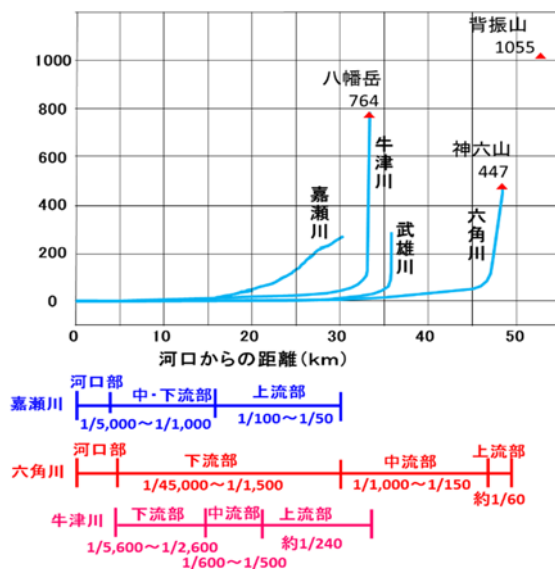
嘉瀬川・六角川の河川縦断面図
